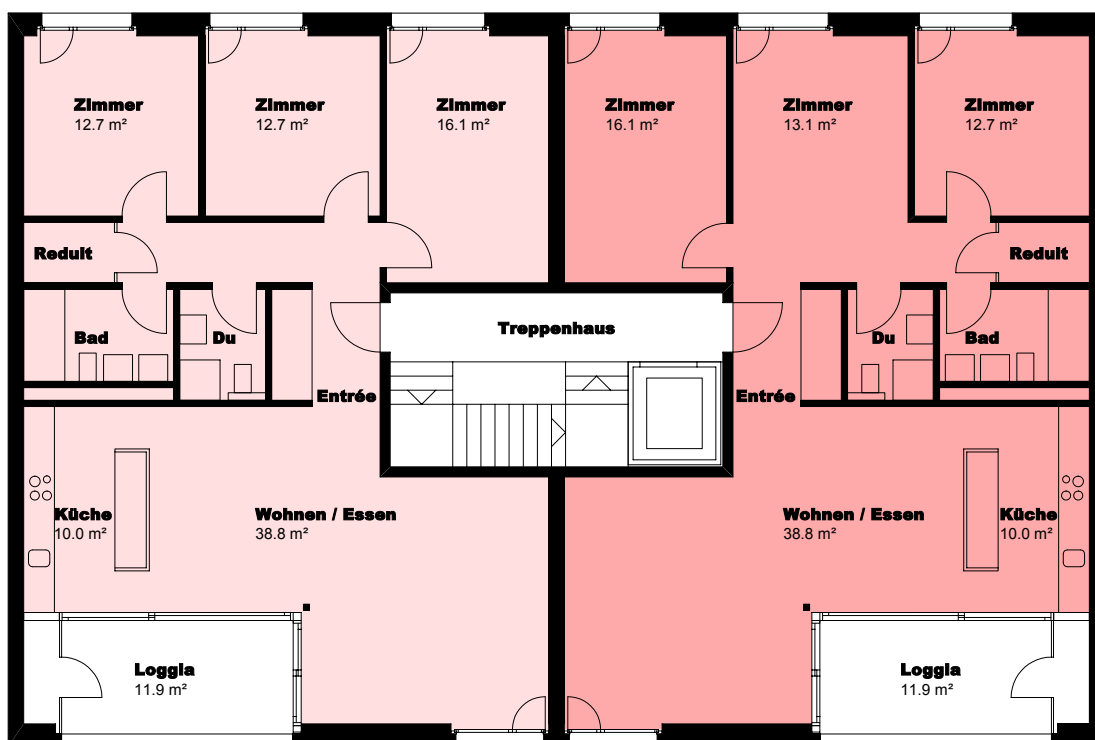
Grundriss M. 1:150
