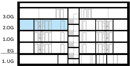
Schnitt
