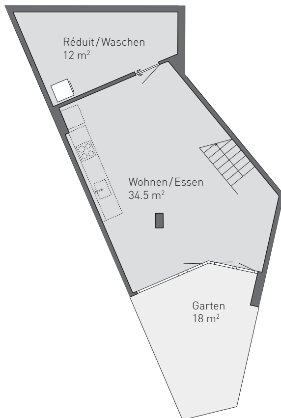
GARTENGESCHOSS
