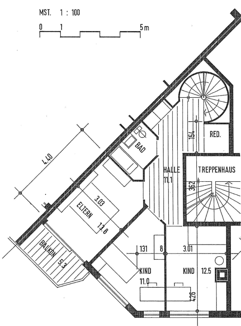
3. OBERGESCHOSS SCHLAFGESCHOSS
