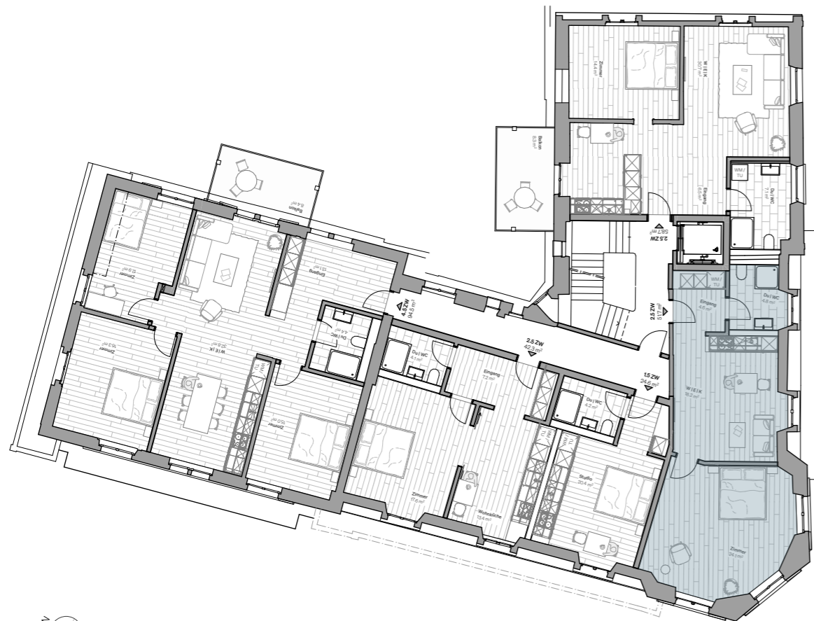
4. Obergeschoss
