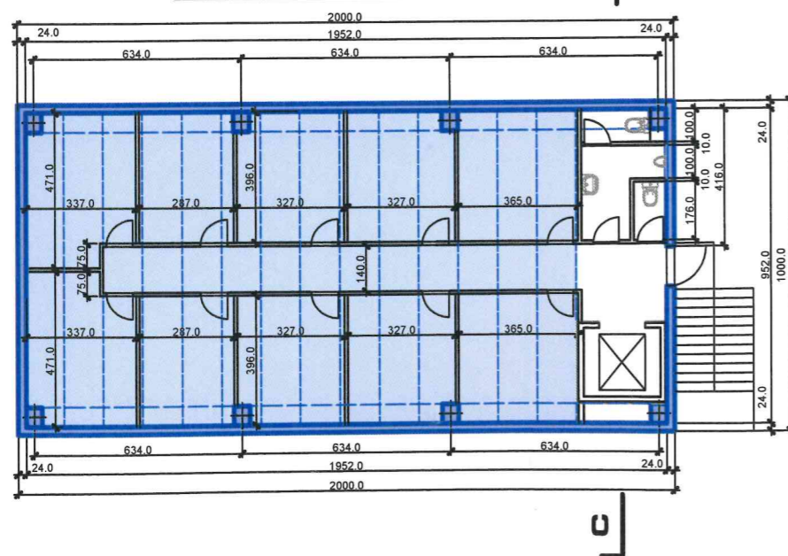
PIANTA PIANO RIALZATO 1:100
