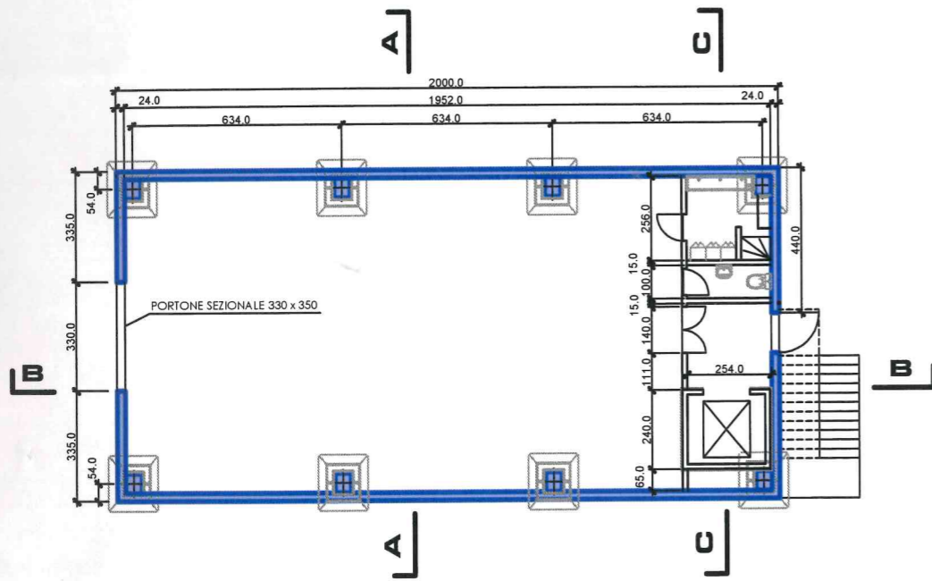
PIANTA PIANO TERRENO 1:100
