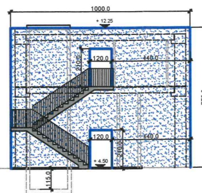
FACCIATA EST 1:100
