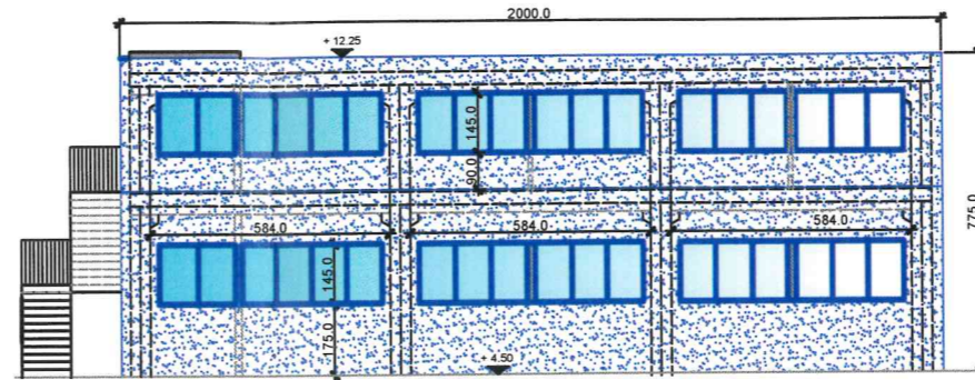
FACCIATA NORD 1:100
