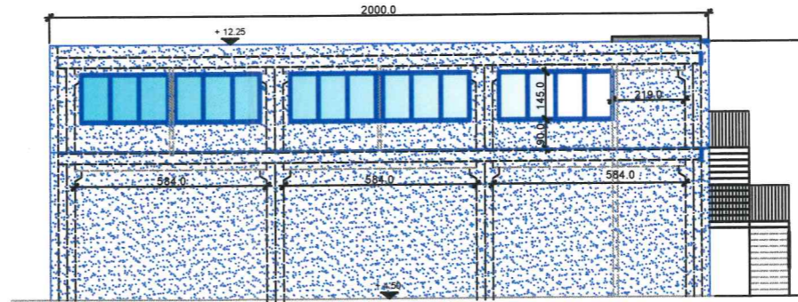
FACCIATA SUD 1:100
