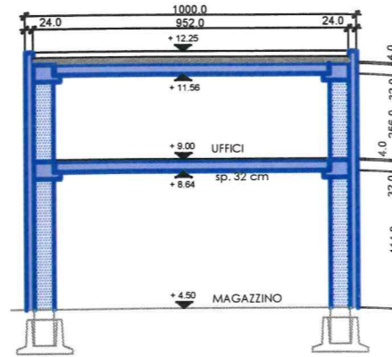
SEZIONE A - A 1:100
