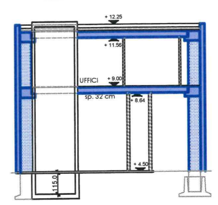
SEZIONE C - C 1:100
