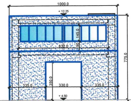
FACCIATA OVEST 1:100
