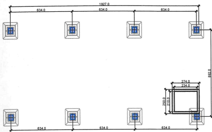
PIANTA FONDAZIONI 1:100
