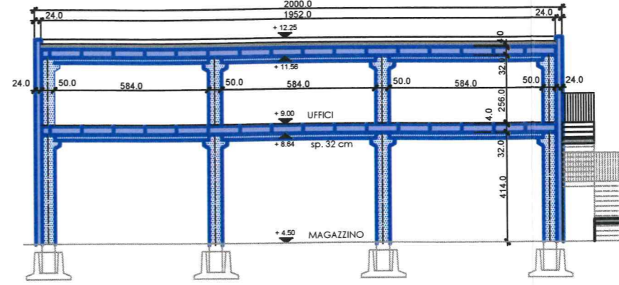
SEZIONE B - B 1:100
