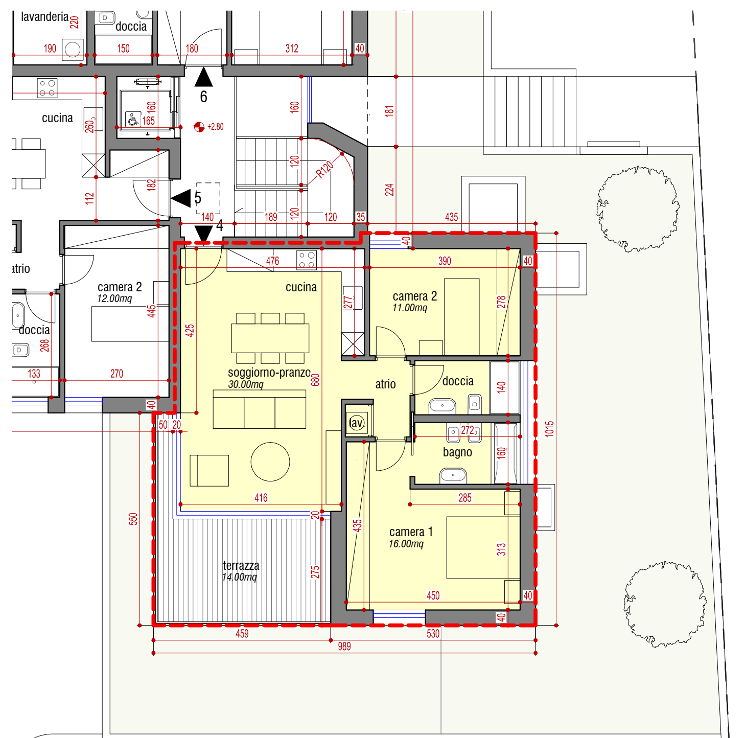
Primo Piano 1:100
