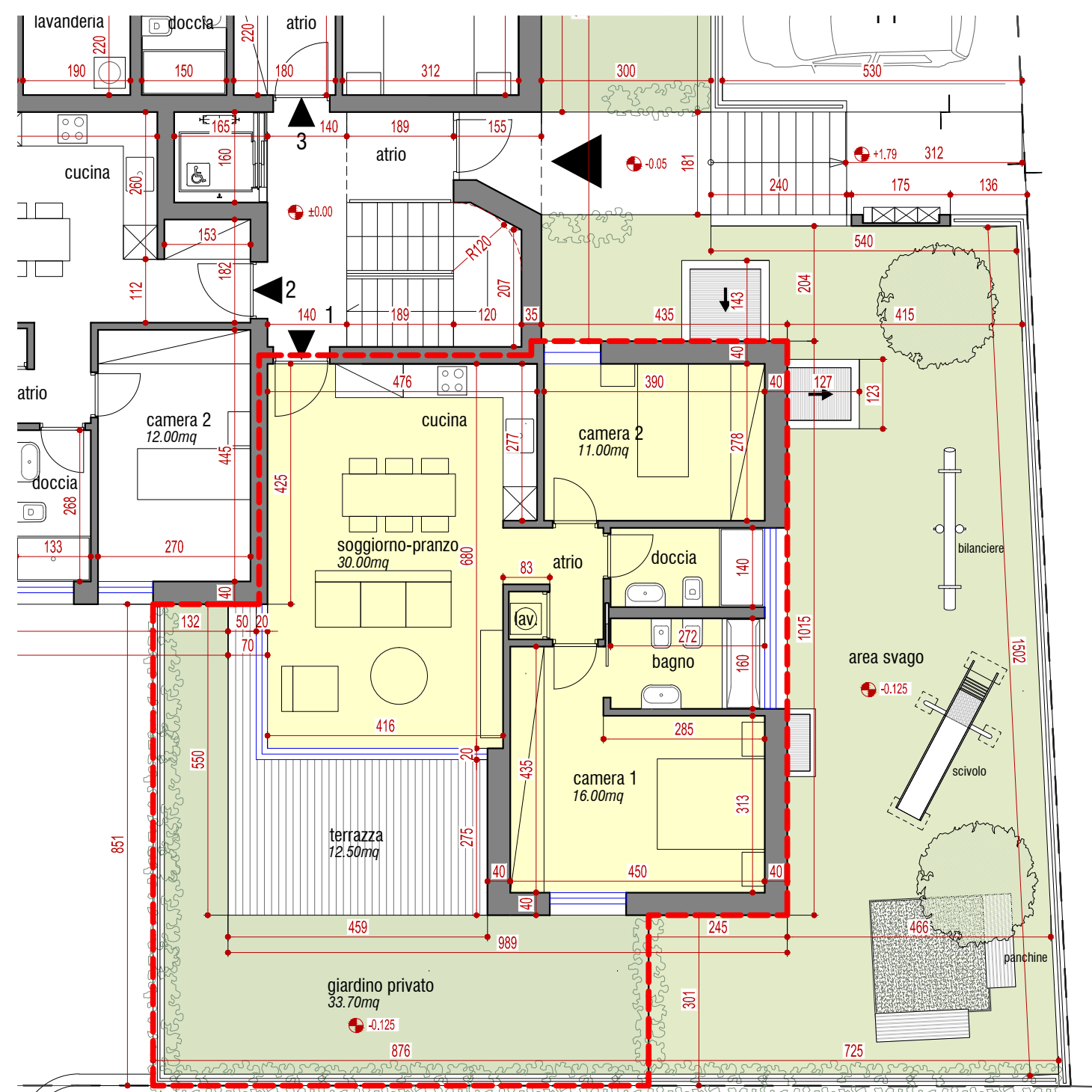
Pianterreno 1:100
