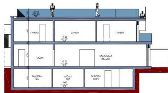
SEZIONE BB
