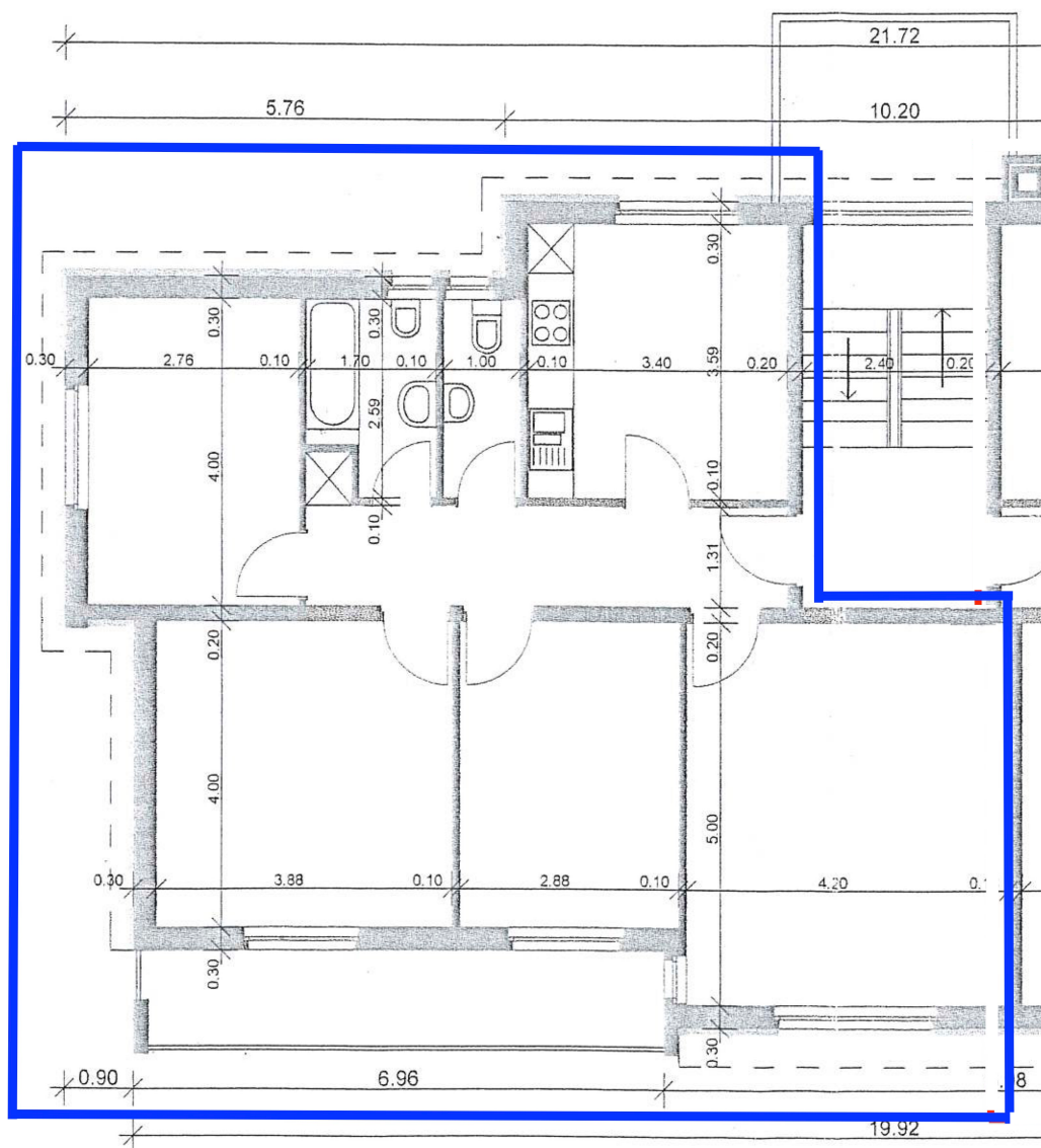
Planimetria appartamento 4.5 locali
