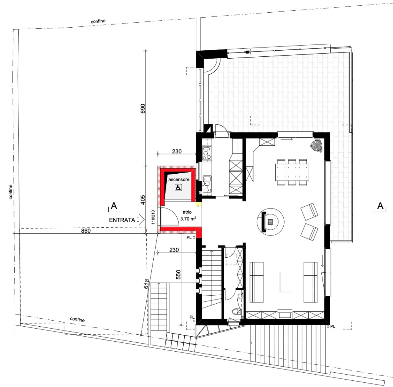
PIANTA PIANO RIALZATO
