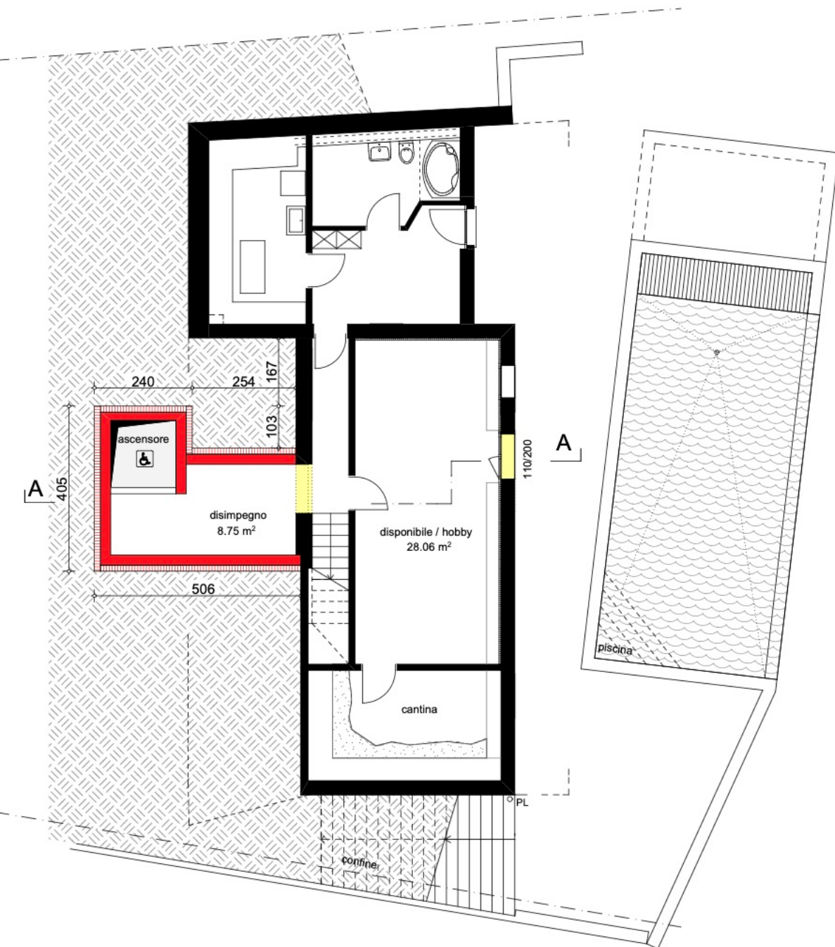
PIANTA PIANO CANTINA
