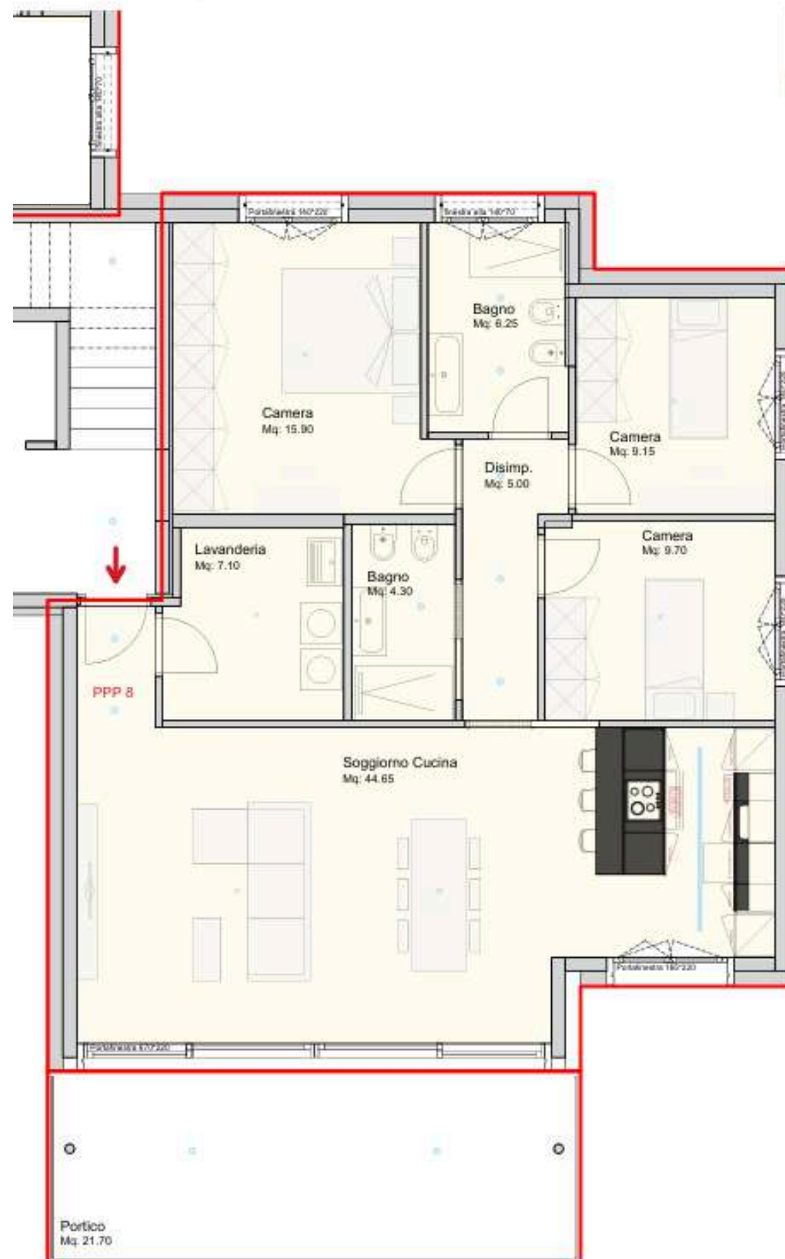
APPARTAMENTO PP8
