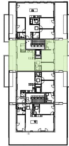
Übersicht Attika
