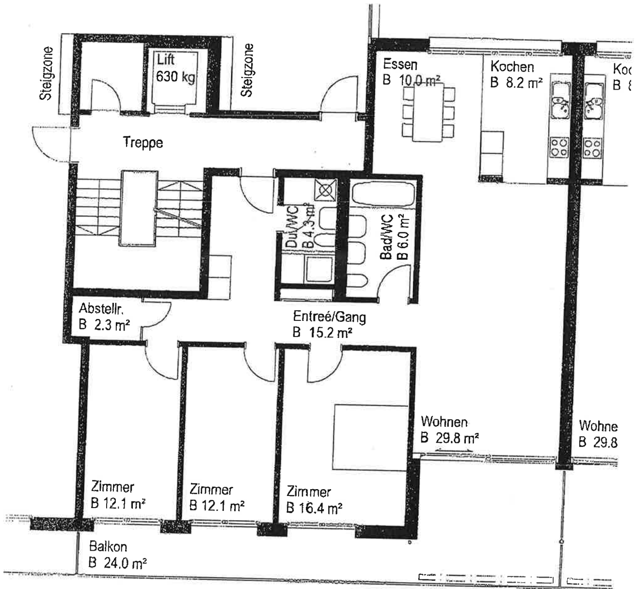
4 1/2 Zimmer-Wohnung Nr. 1112 + 1122 NWF 116.4 m 2
