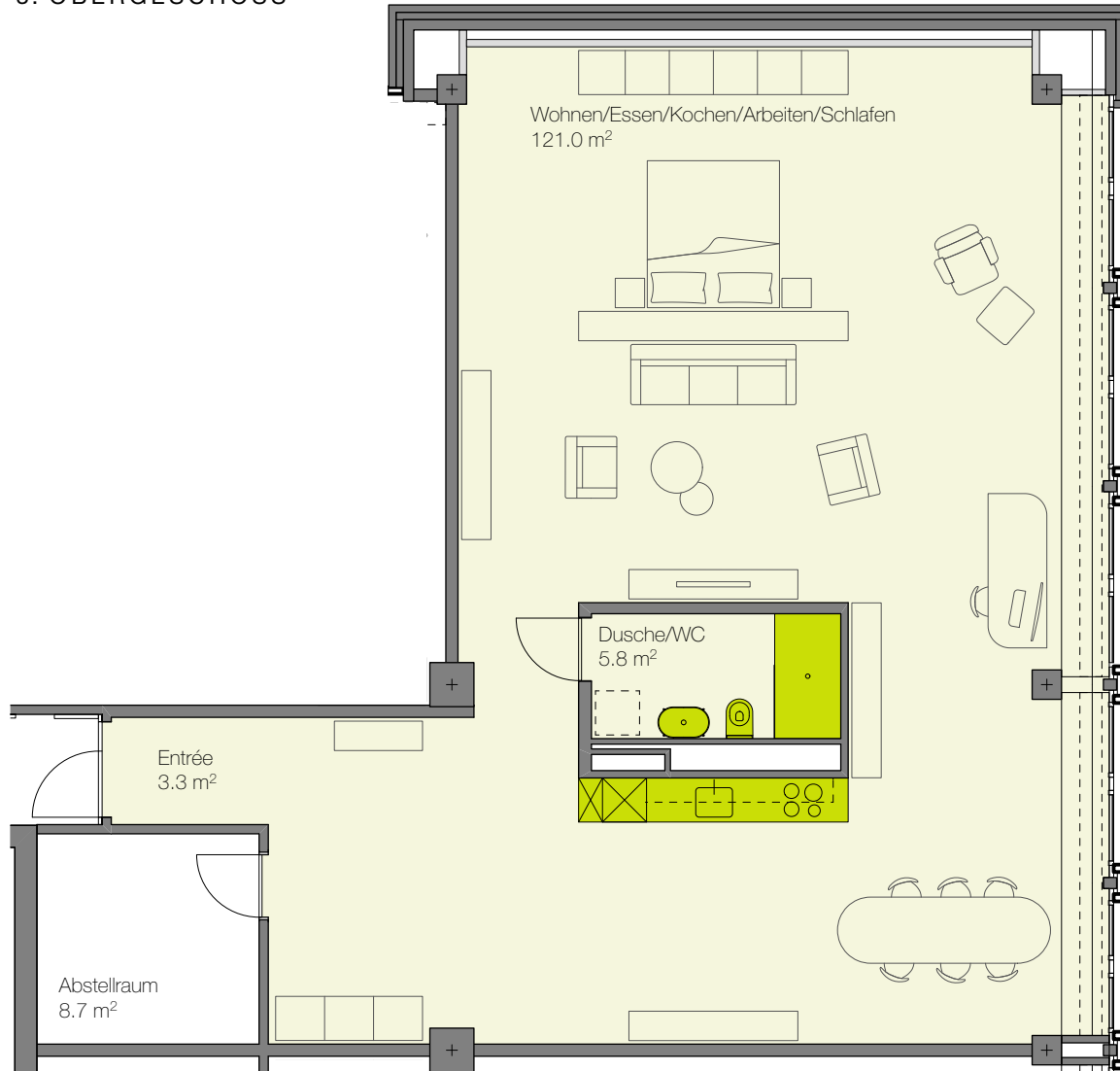
Grundriss 3. Obergeschoss M 1:100
