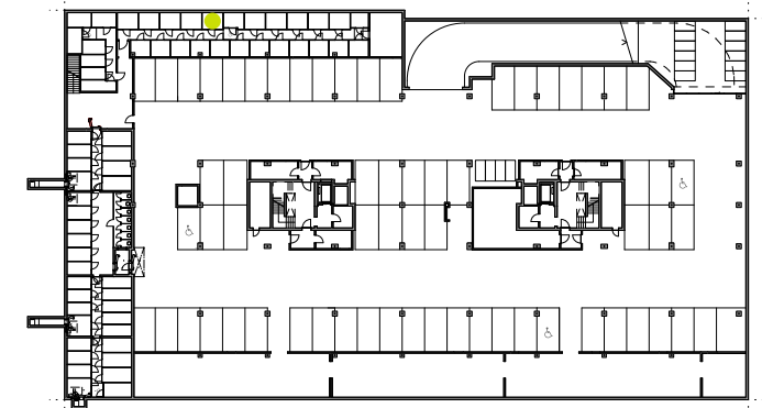
Grundriss 2. Untergeschoss Mst. 1:1000
