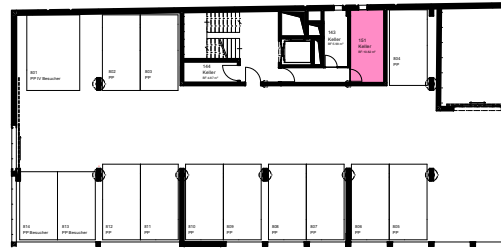
Übersichtsplan -1.UG
