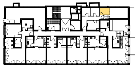
Übersichtsplan EG
