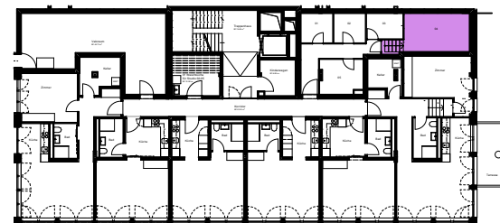
Übersichtsplan EG
