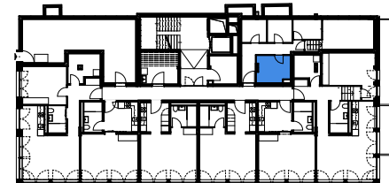
Übersichtsplan EG
