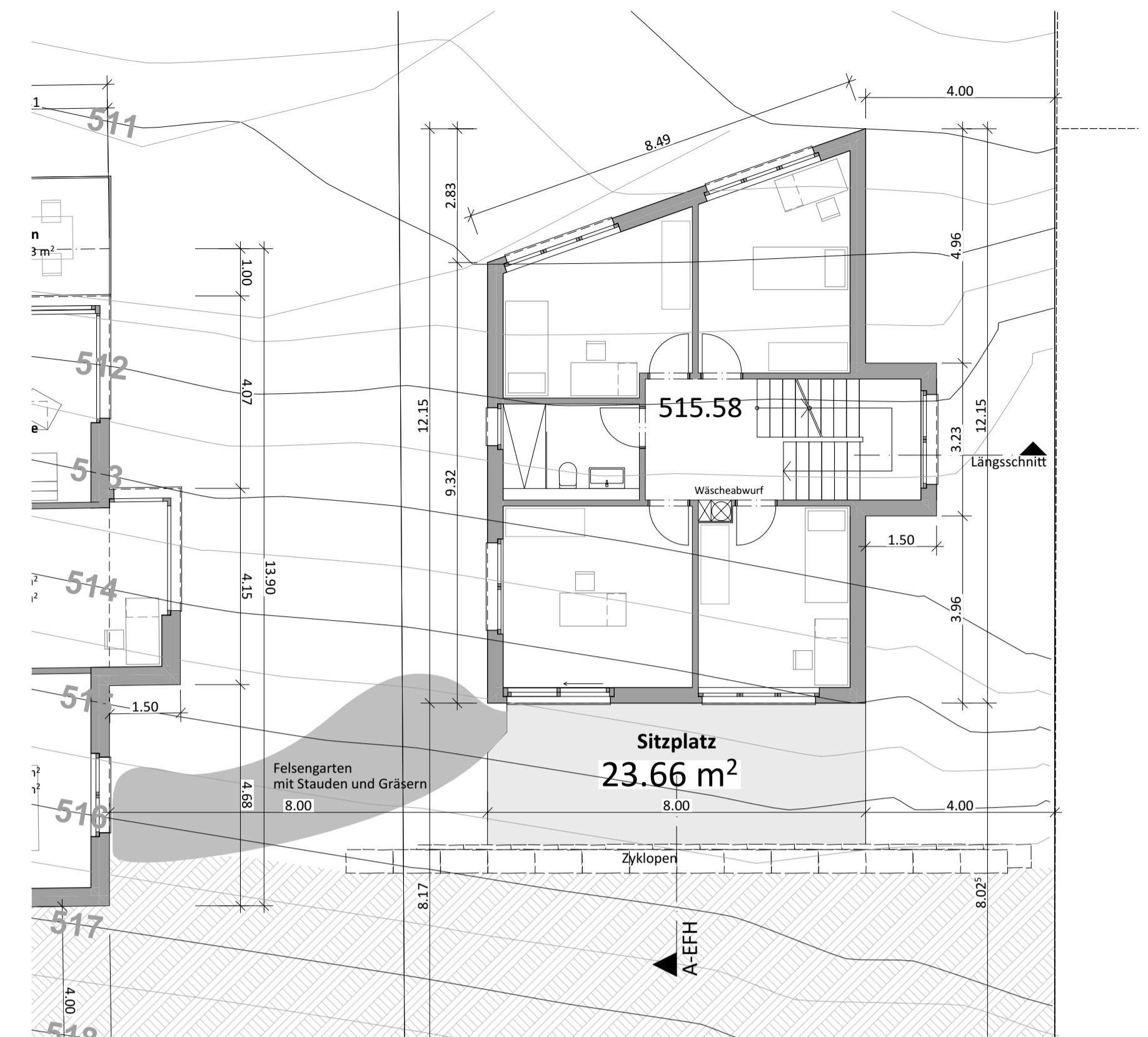
Grundriss 1.OG
