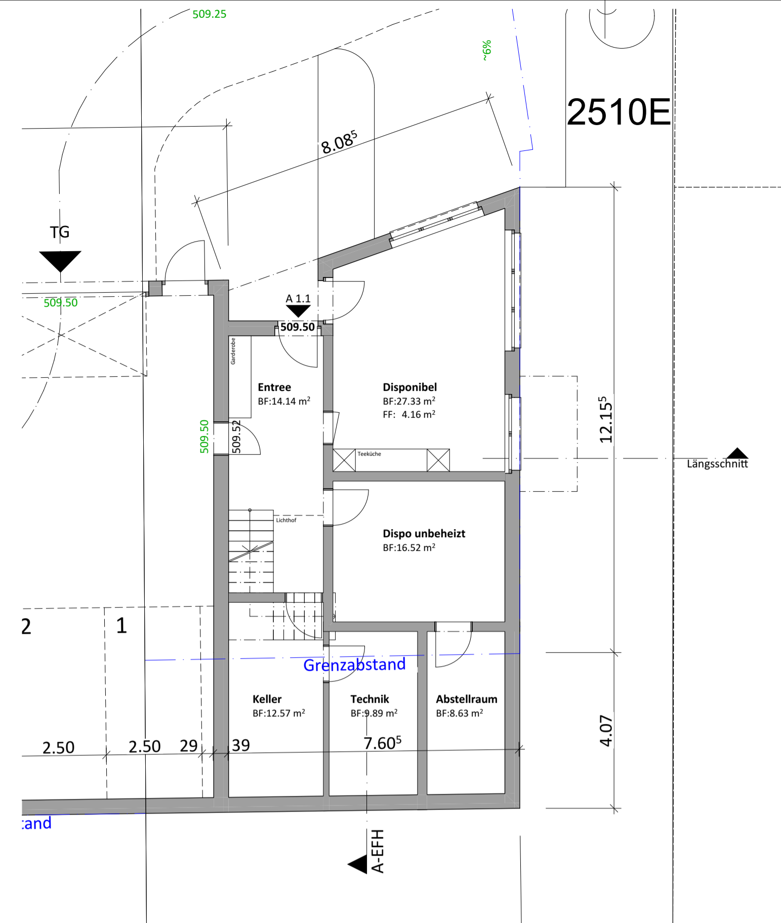
Grundriss UG
