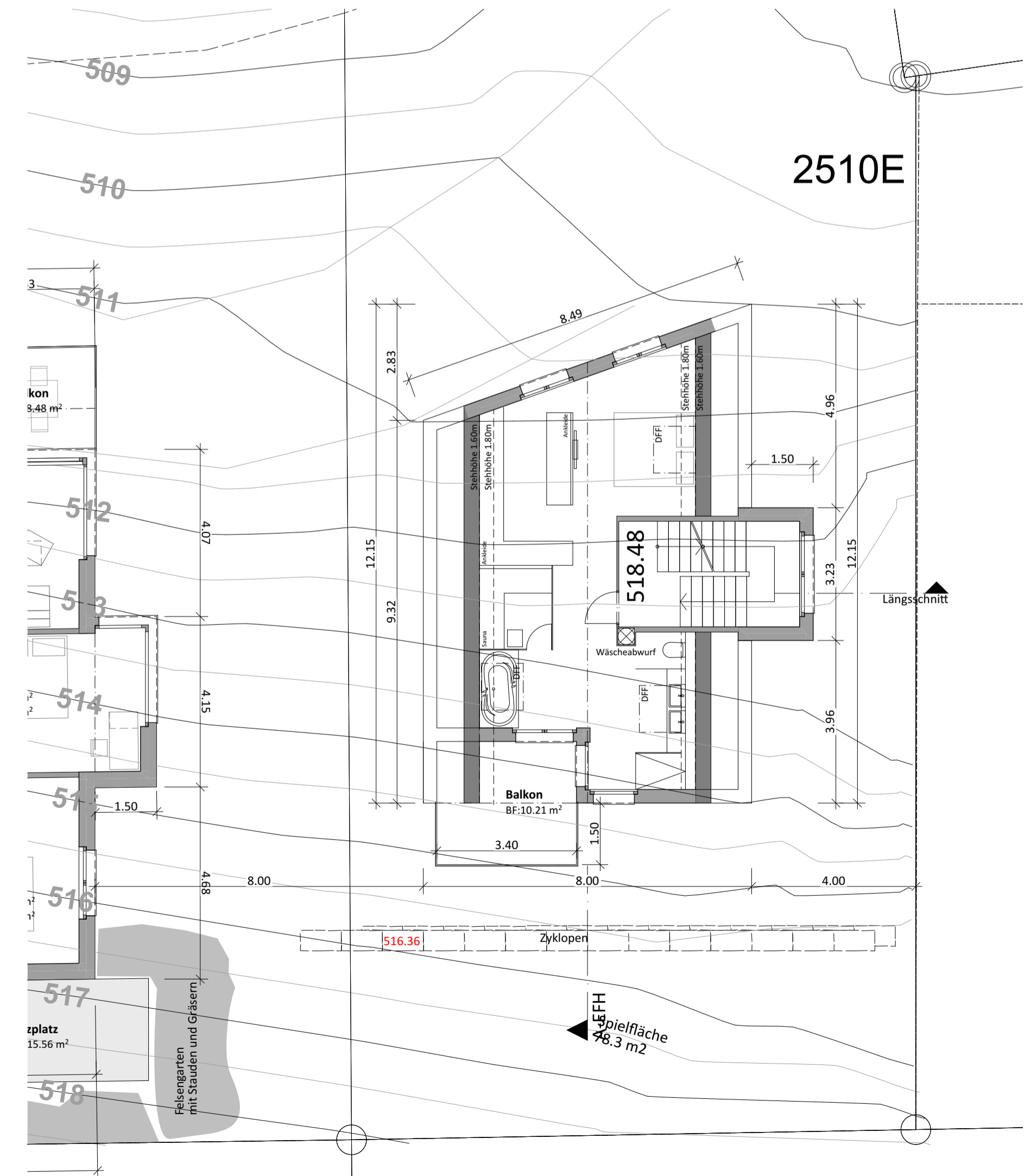
Grundriss 2.OG
