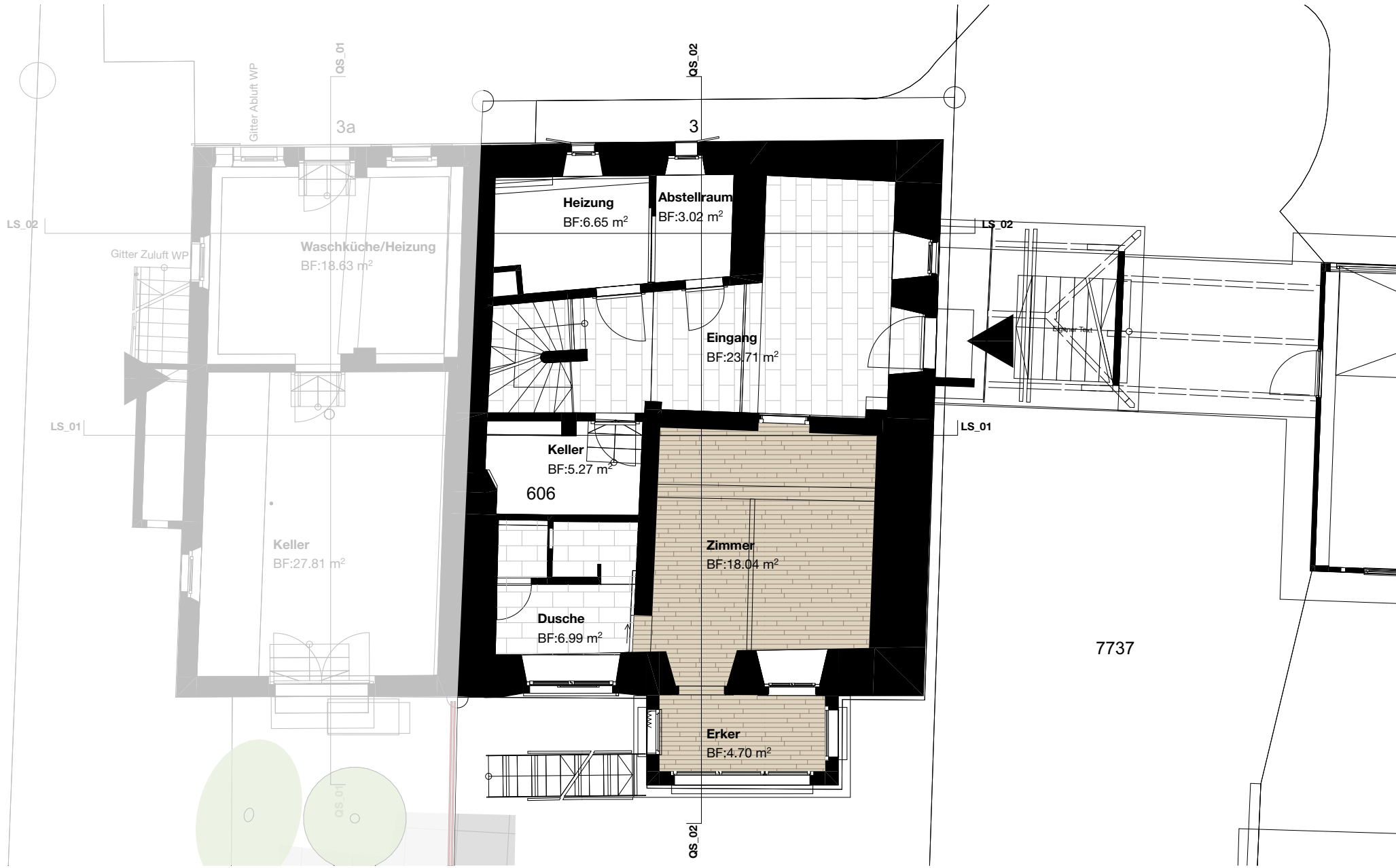
Untergeschoss 1:100 ( Chrummbächliweg 3 )
