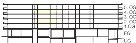
Schnitt
