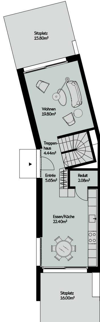
Erdgeschoss
