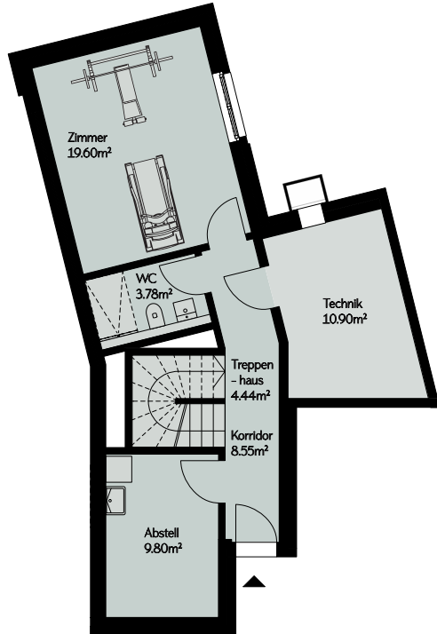
Untergeschoss
