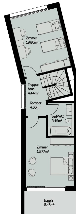
Obergeschoss
