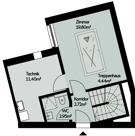
Untergeschoss
