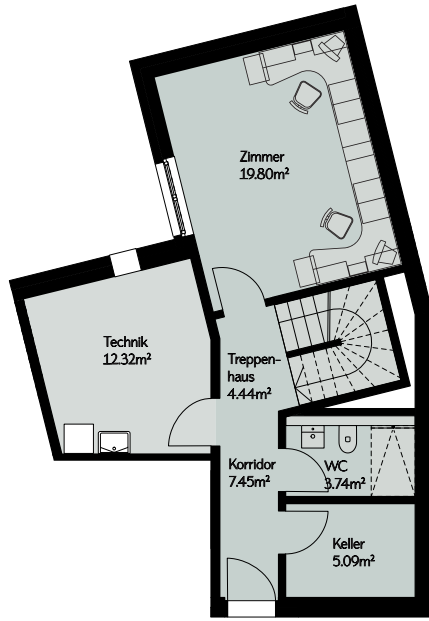
Untergeschoss
