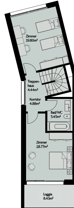
Obergeschoss
