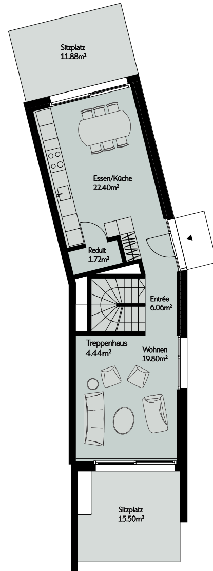
Erdgeschoss
