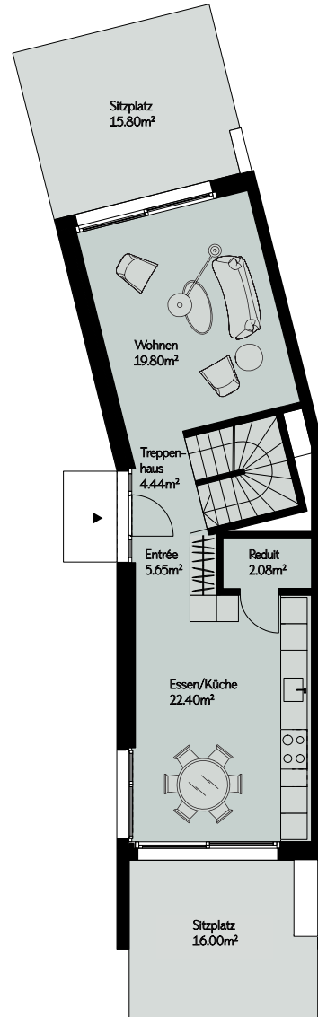
Erdgeschoss
