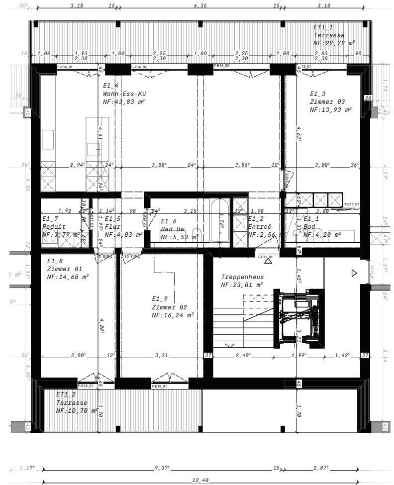
Grundriss OG
