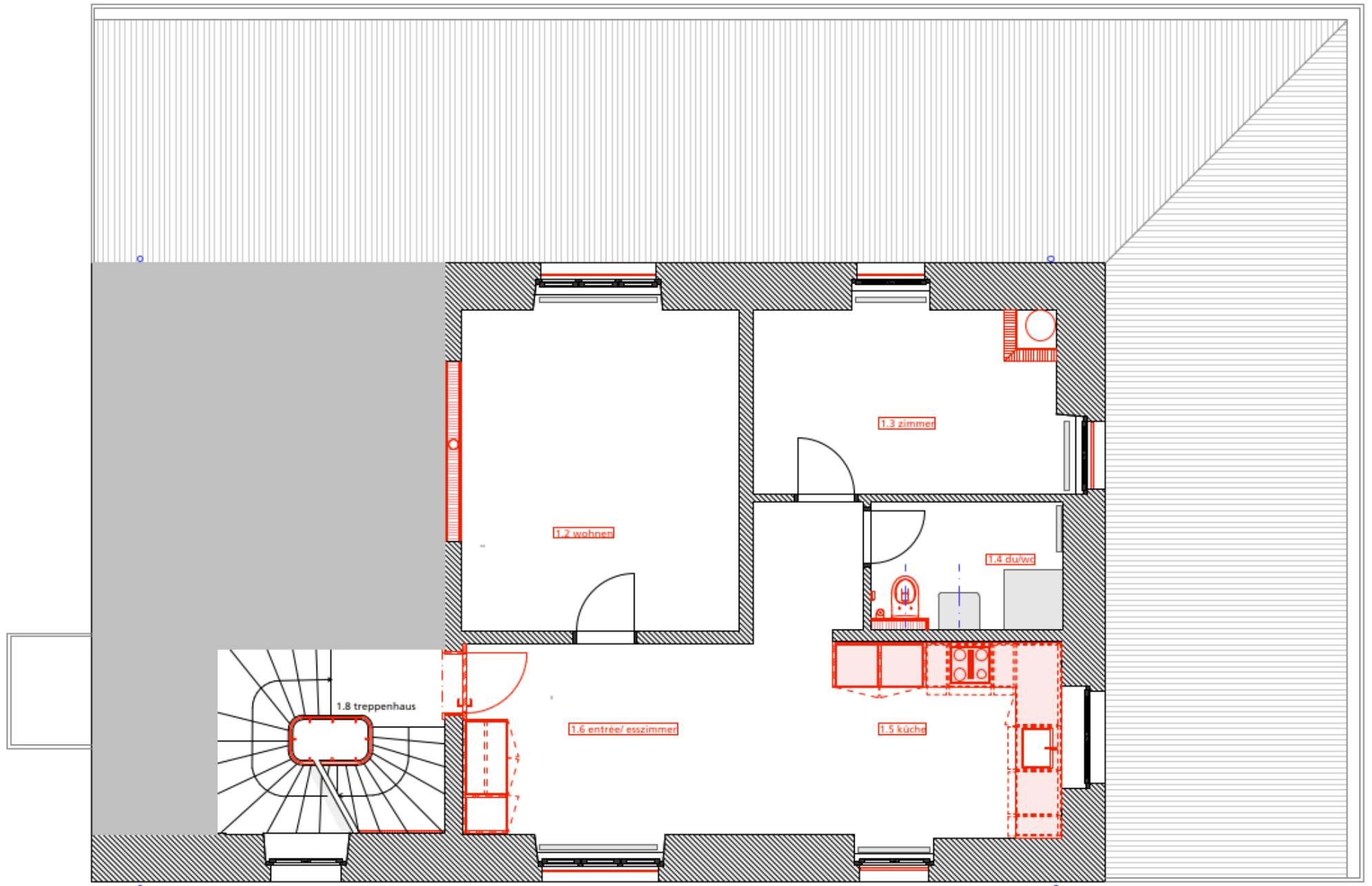
grundriss 1. obergeschoss
