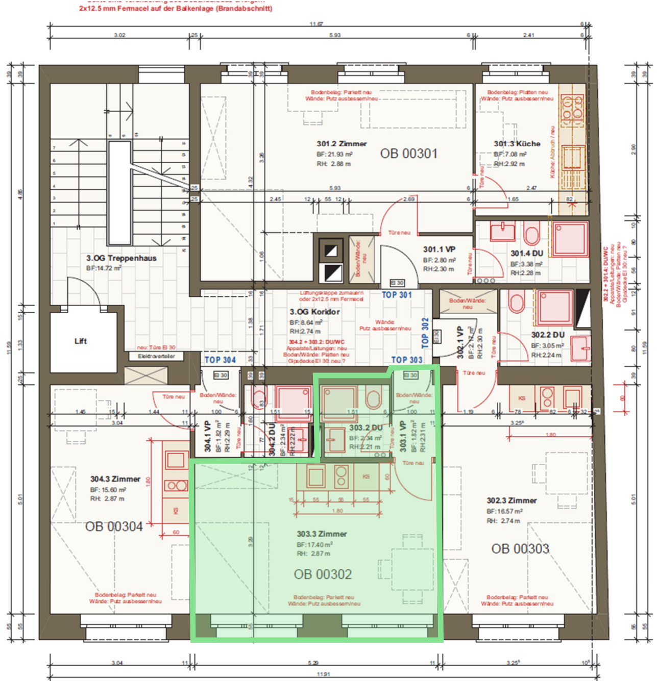
3. Obergeschoss
