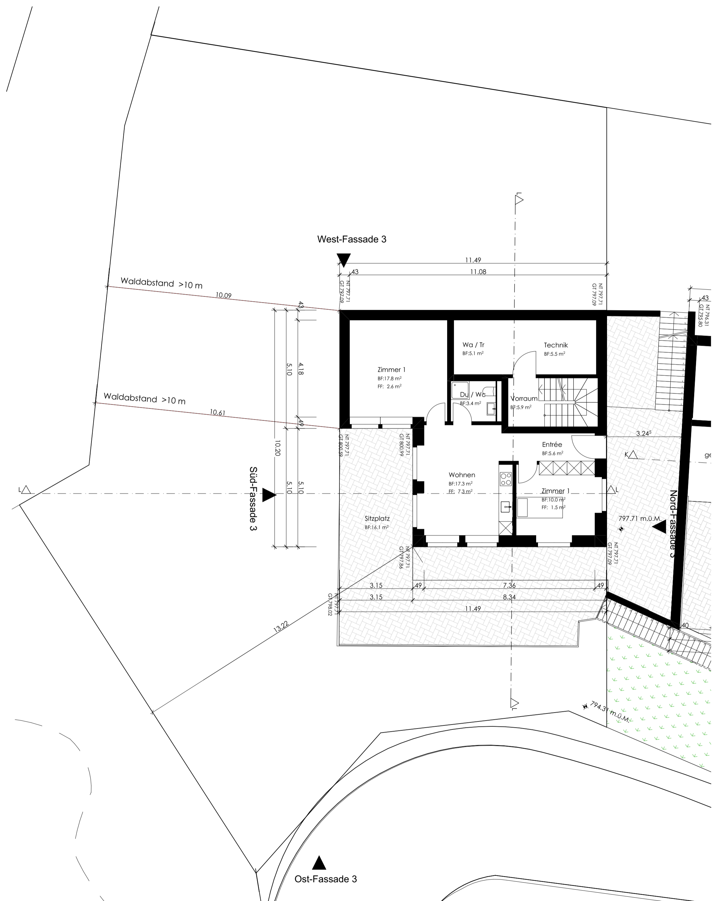
M01 Untergeschoss
