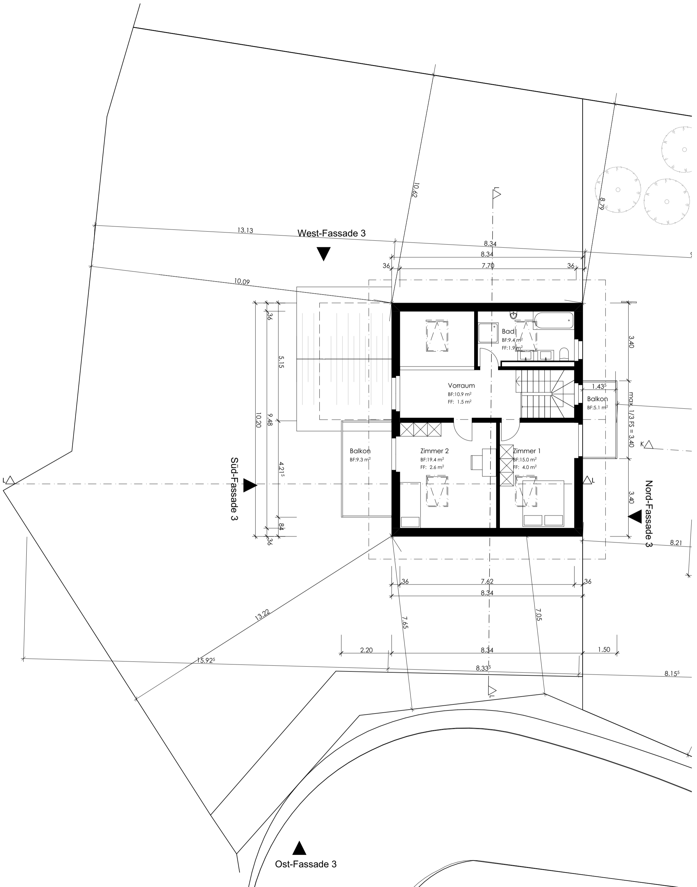
P01 Obergeschoss
