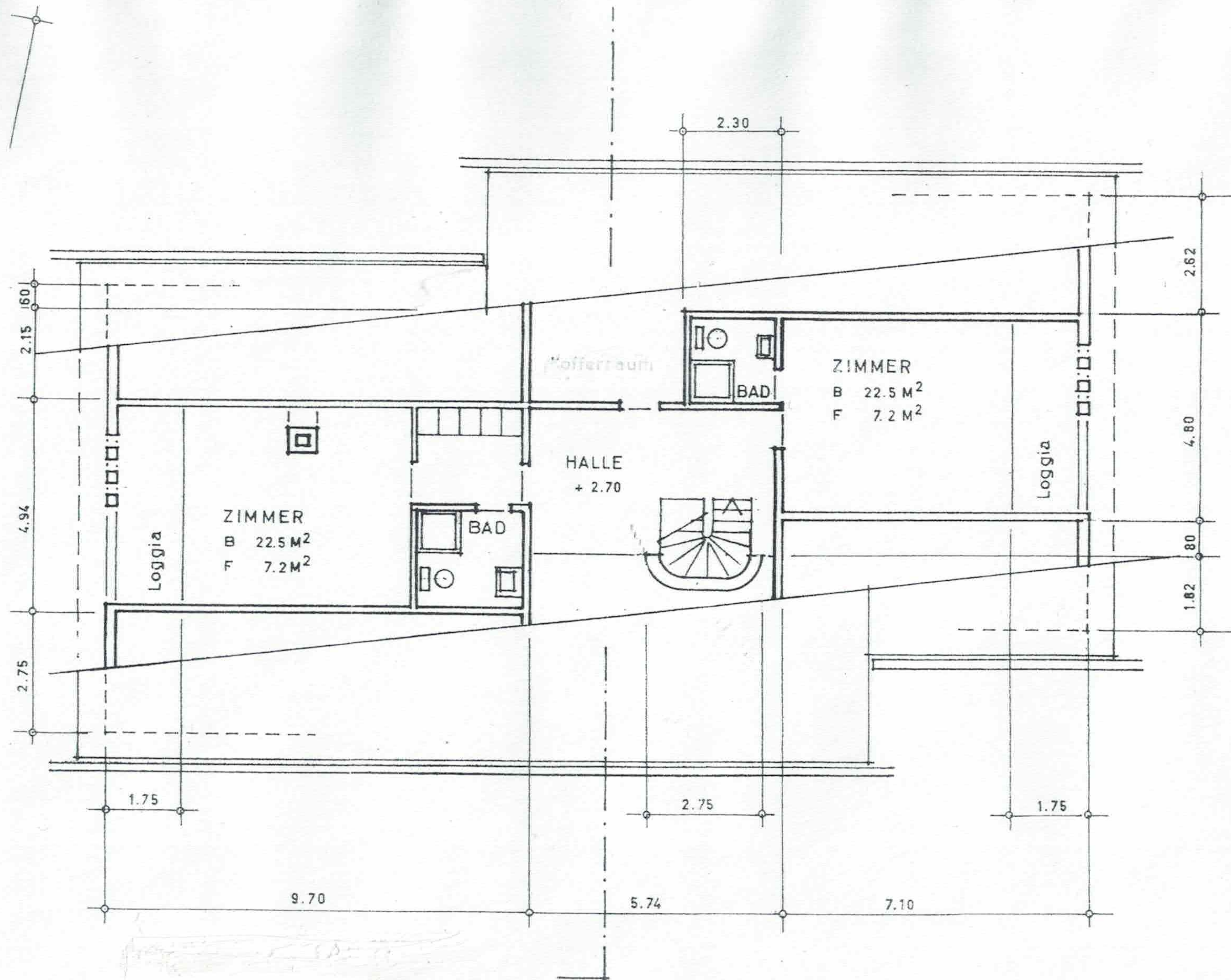
Grundriss Dachgeschoss
