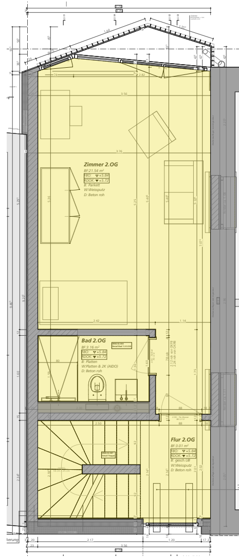
2. OBERGESCHOSS
