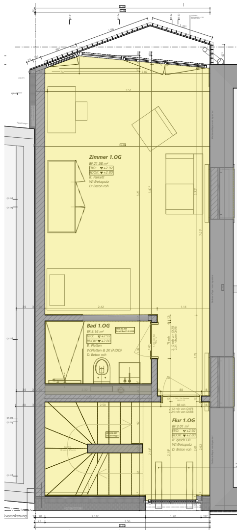
1. OBERGESCHOSS
