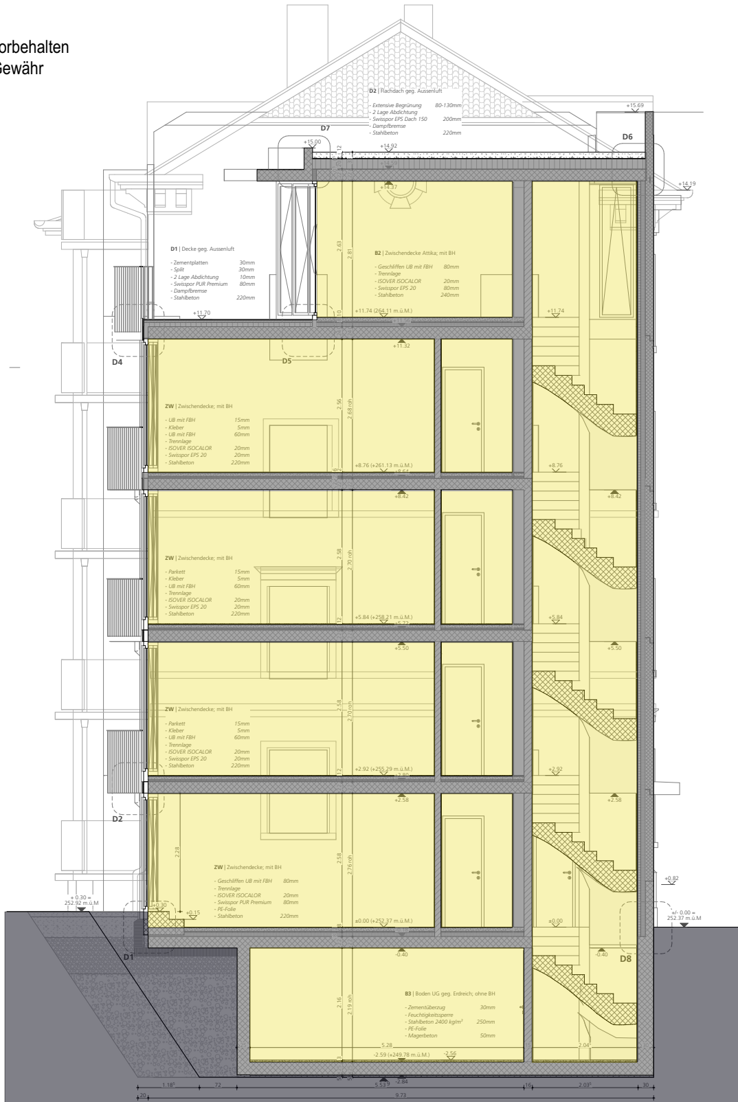
SCHNITT LÄNGS
