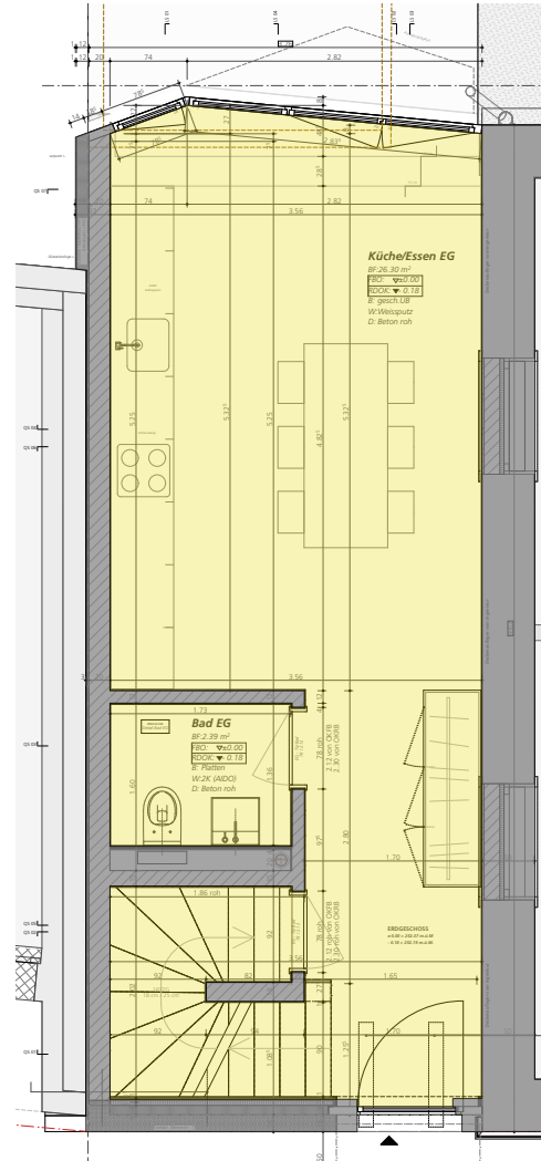
ERDGESCHOSS
