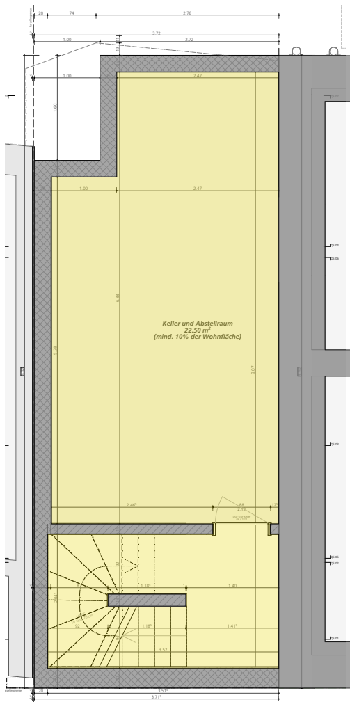
UNTERGESCHOSS
