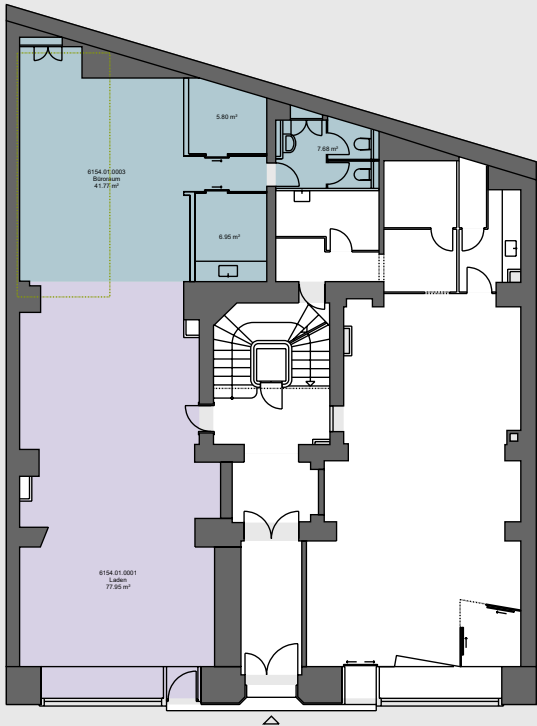
Erdgeschoss
