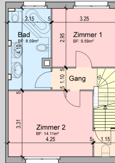
Obergeschoss
