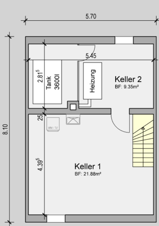
Untergeschoss
