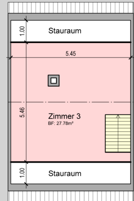
Dachgeschoss
