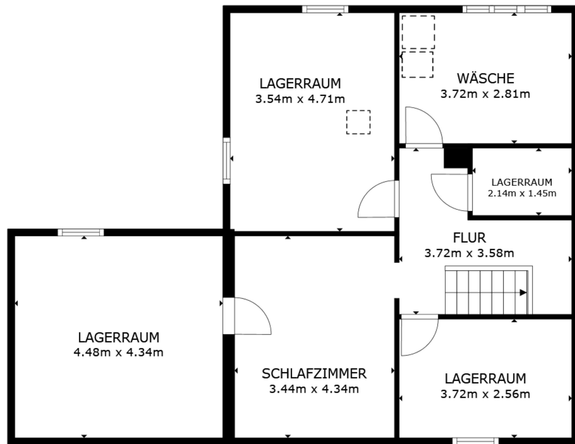
STOCKWERK 1
