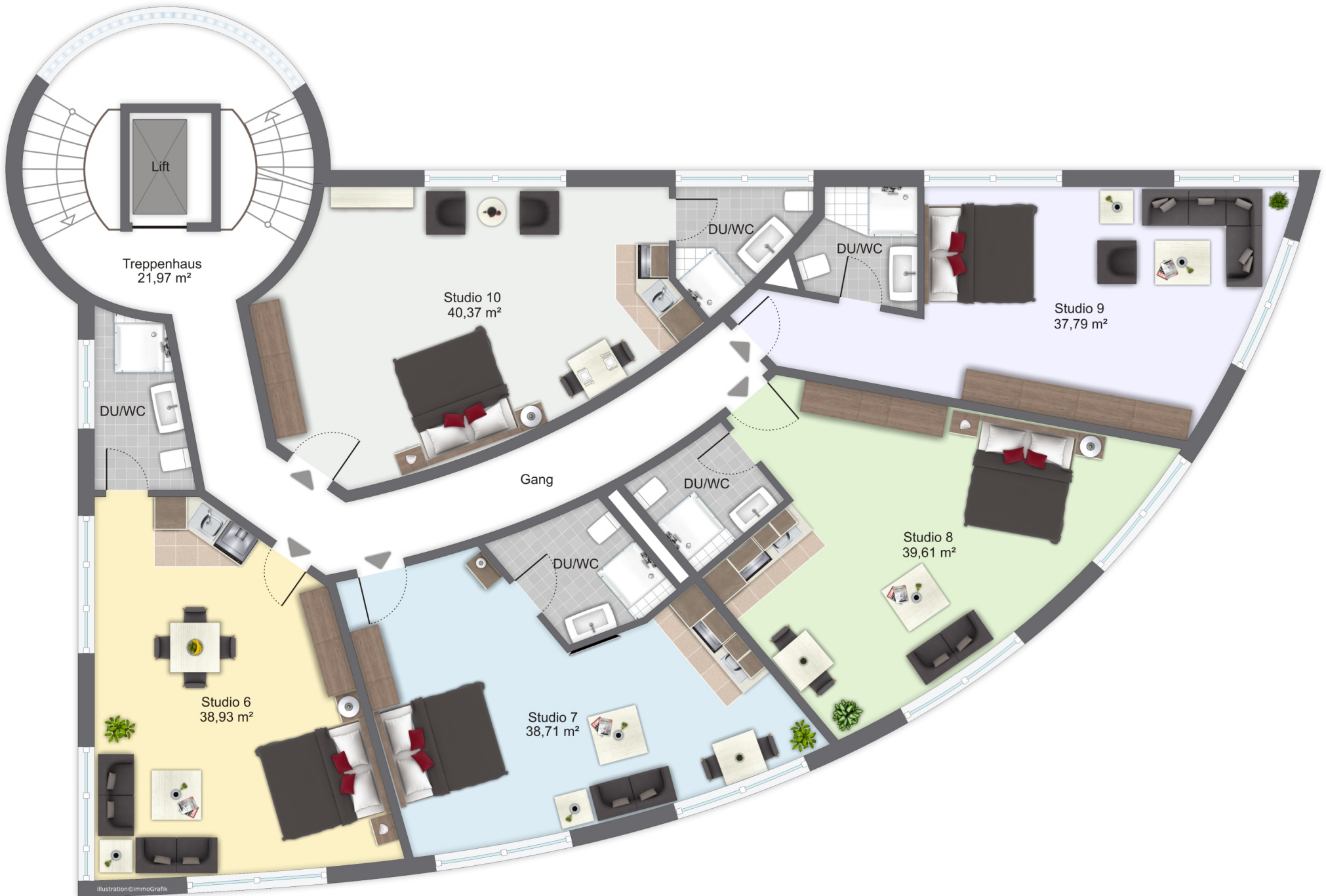
1. Obergeschoss - Studio 6 - 10
