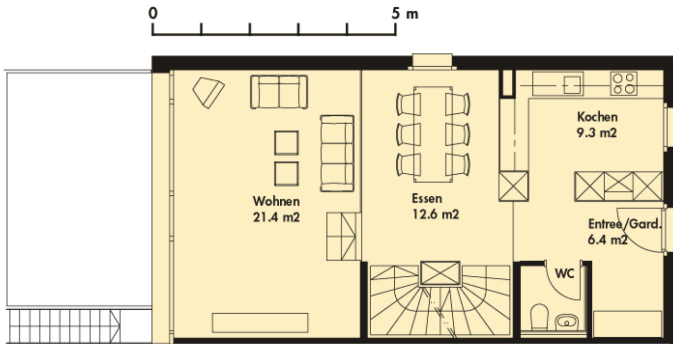
Erdgeschoss
