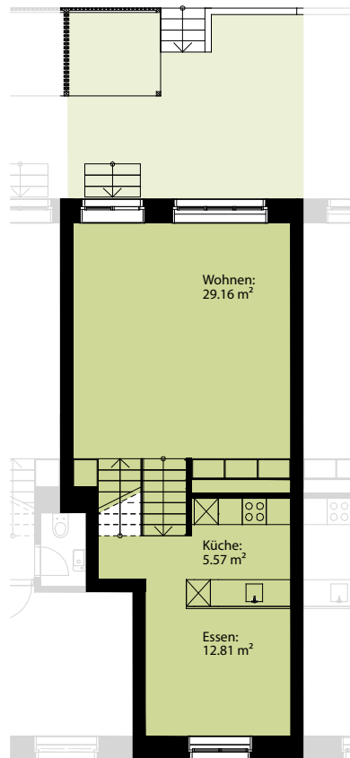
1. Obergeschoss
