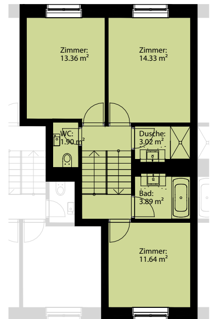
2. Obergeschoss
