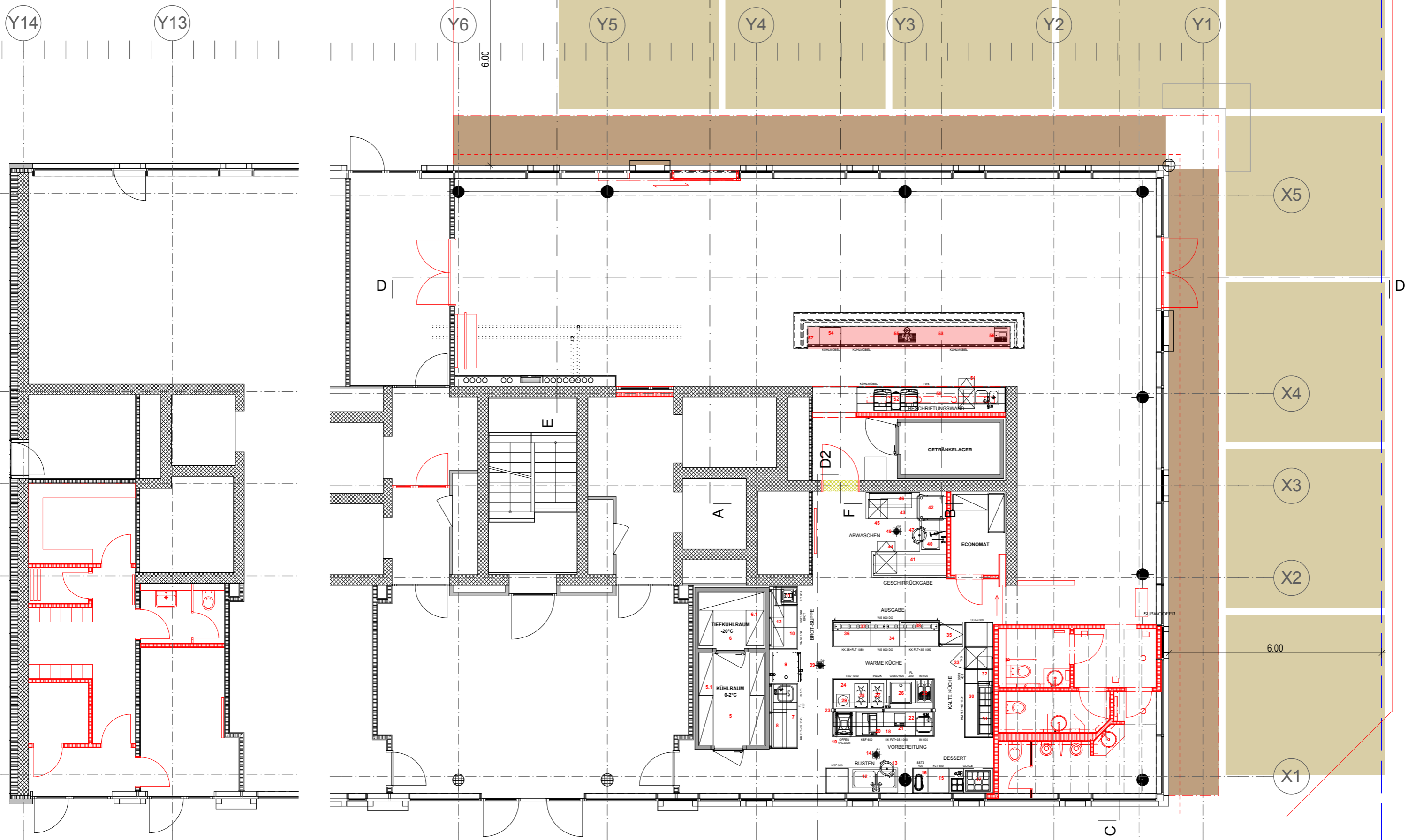
GRUNDRISS EG
