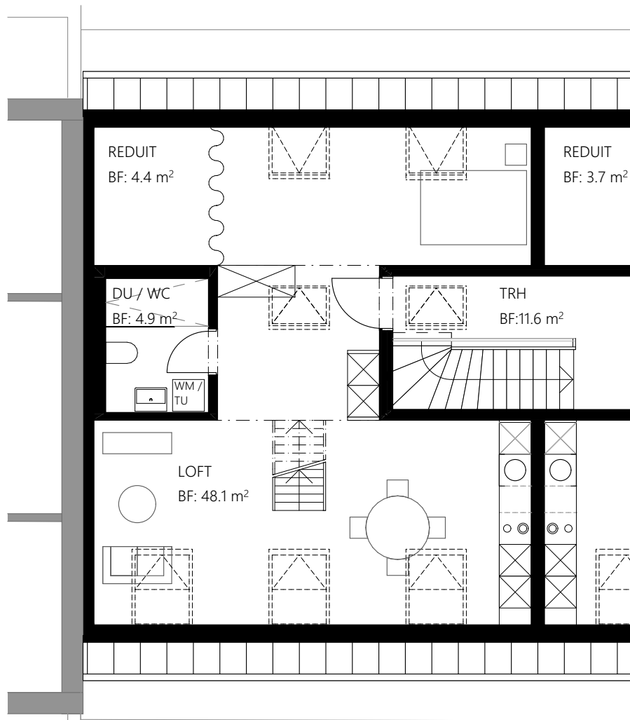
GRUNDRISS ATTIKA 2 FLÄCHE: 57.40M 2 WOHNUNG 1 FLÄCHE TOTAL: 69.70M 2
