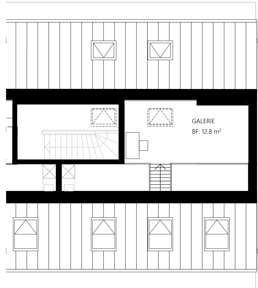
GRUNDRISS GALERIE FLÄCHE: 12.80M 2
