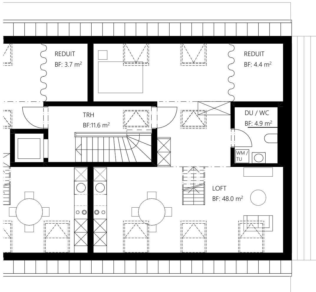
GRUNDRISS ATTIKA 2 FLÄCHE: 57.30M 2 WOHNUNG 4 FLÄCHE TOTAL: 70.10M 2
