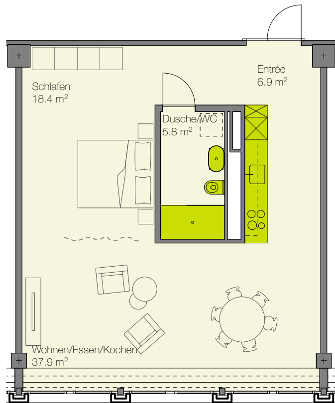
Grundriss 1. Obergeschoss Mst. 1:100
