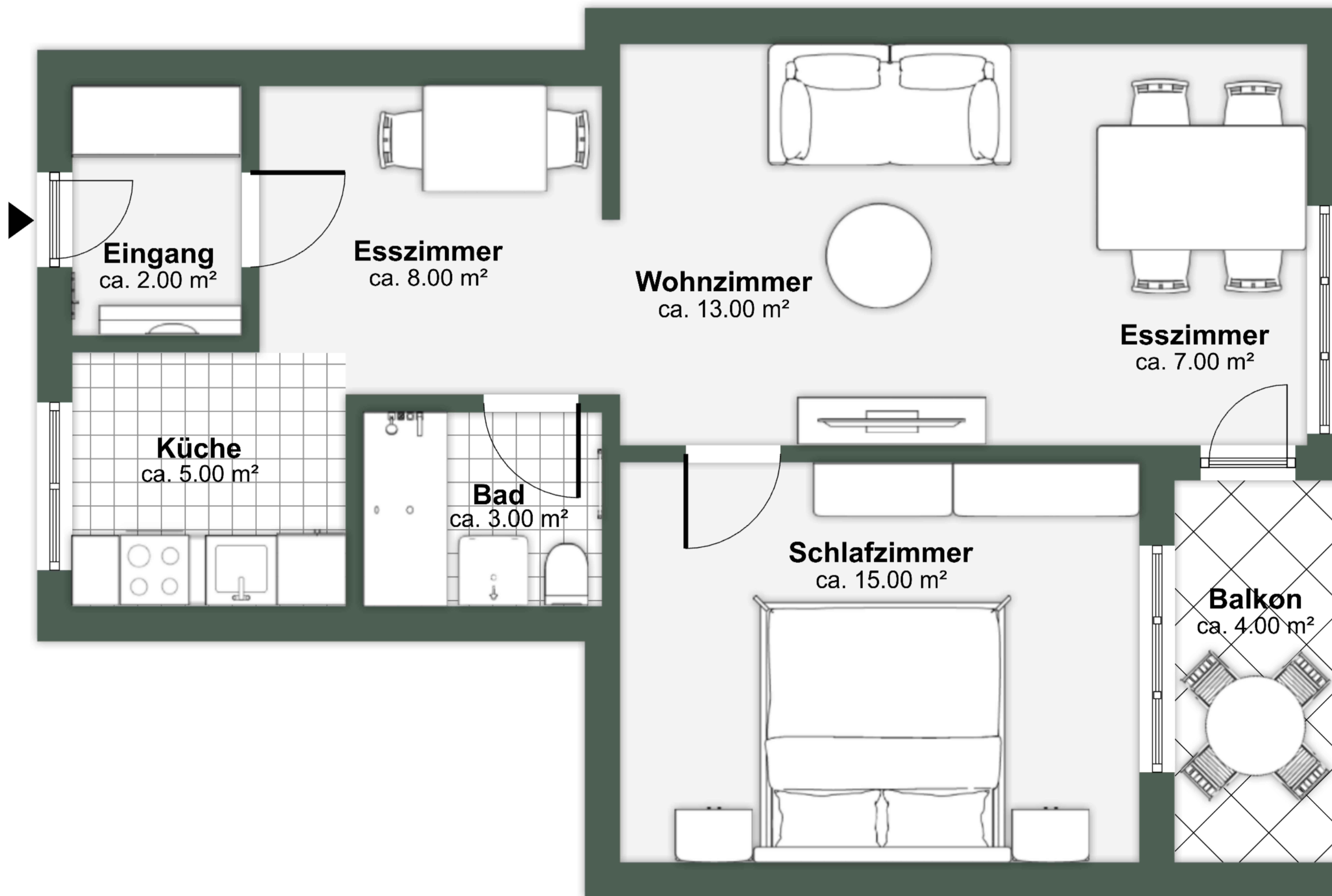
1. Obergeschoss
