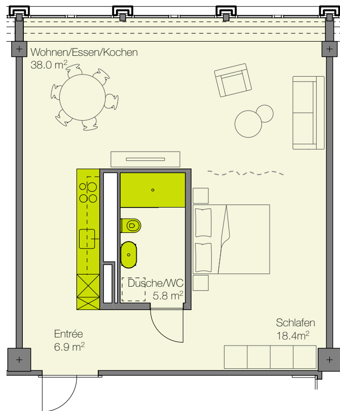
Grundriss 3. Obergeschoss Mst. 1:100
