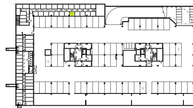
Grundriss 2. Untergeschoss Mst. 1:1000
