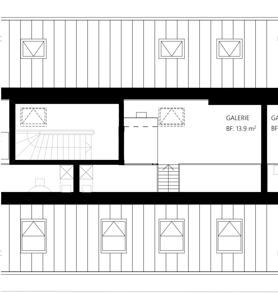
GRUNDRISS GALERIE FLÄCHE: 13.90M²
