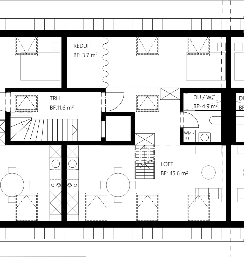
GRUNDRISS ATTIKA 2 FLÄCHE: 54.20M² WOHNUNG 2 FLÄCHE TOTAL: 68.10M²
