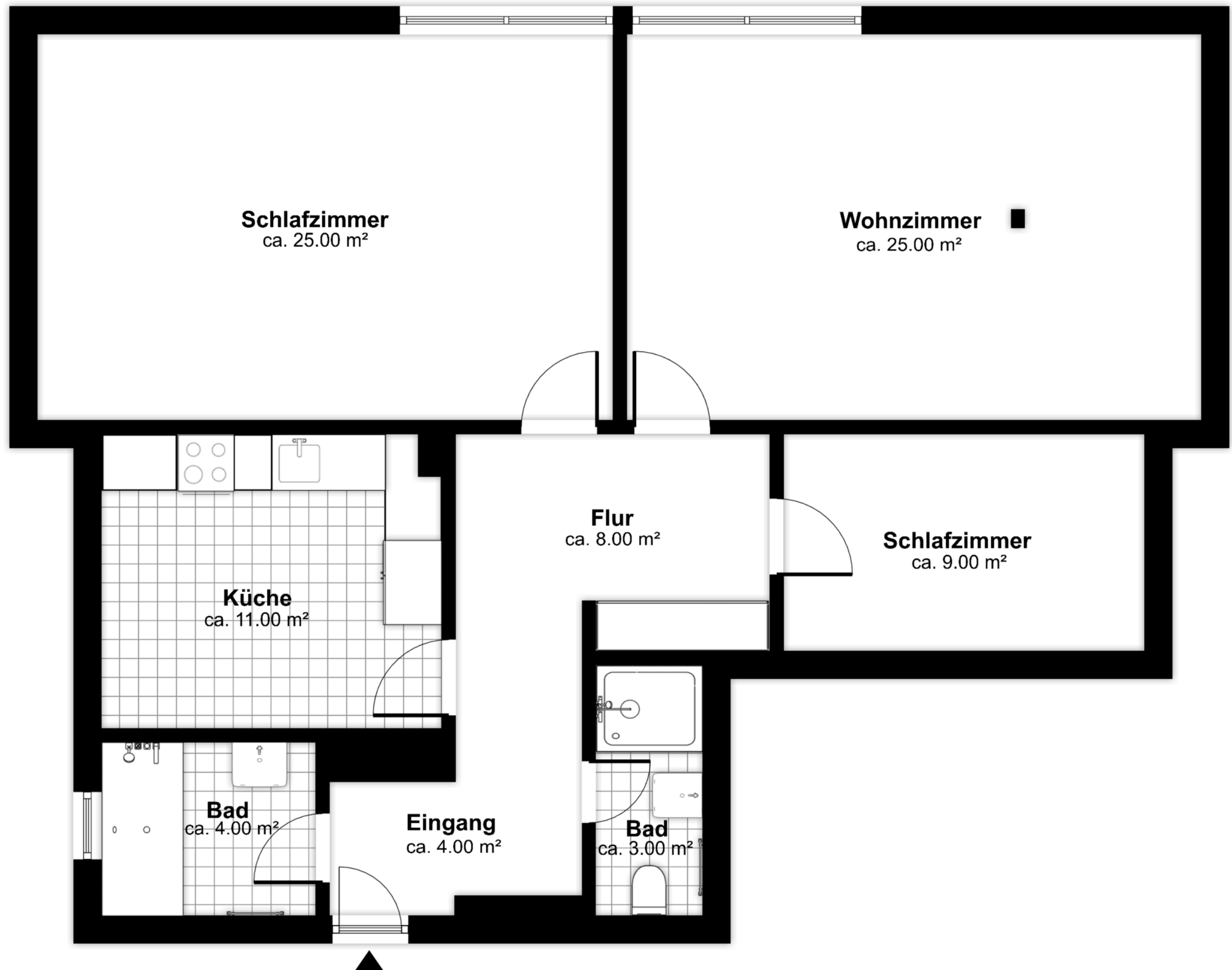
1. Obergeschoss
