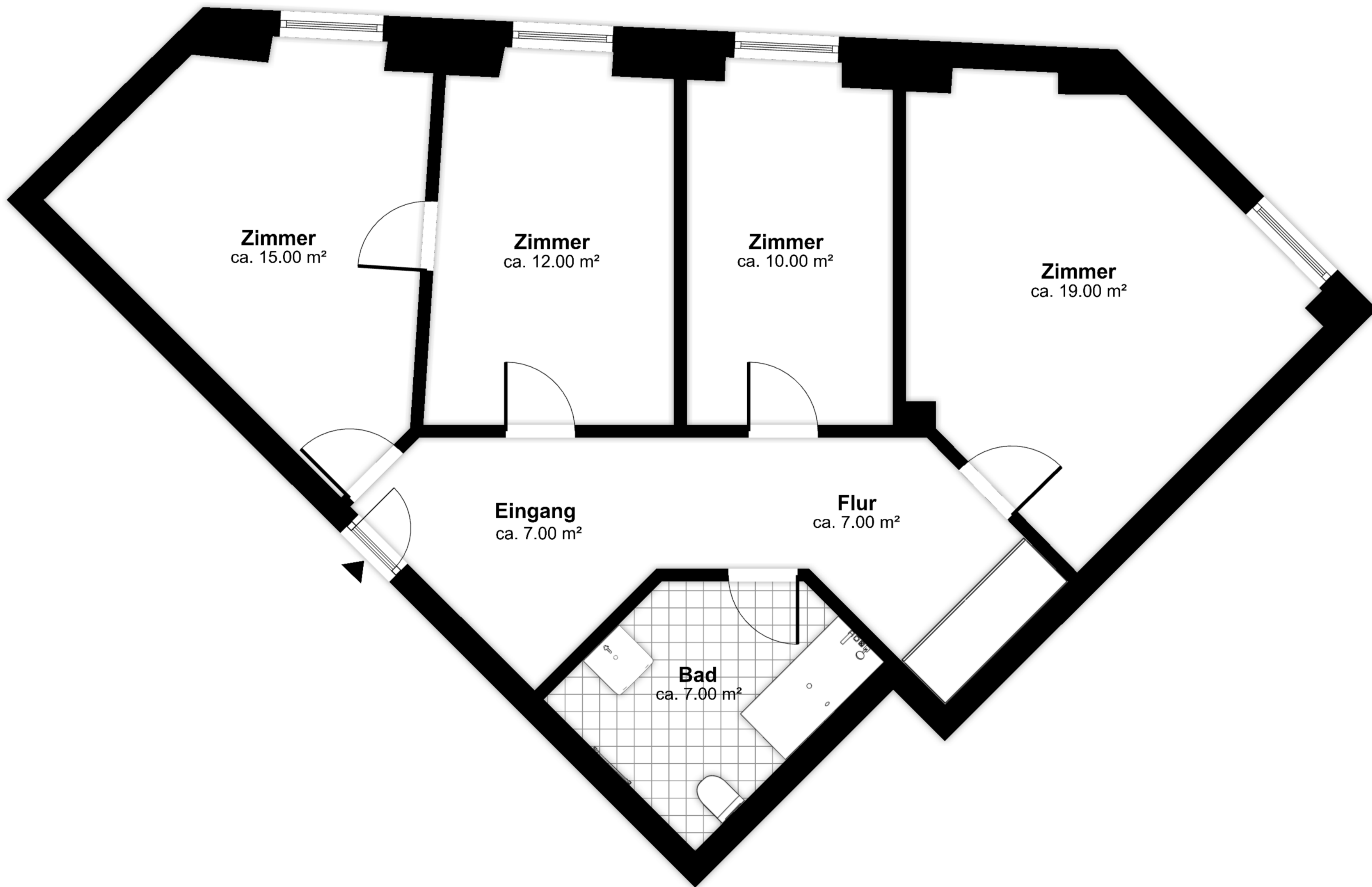
1. Obergeschoss
