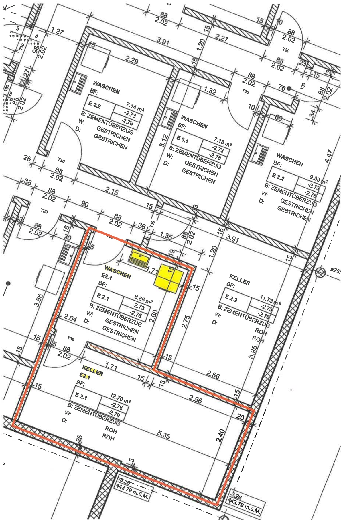
ÜBERBAUUNG SONNENBÜHL DIETLIKON, KELLER/WASCHEN E2.1, 1:50, 10.06.04
