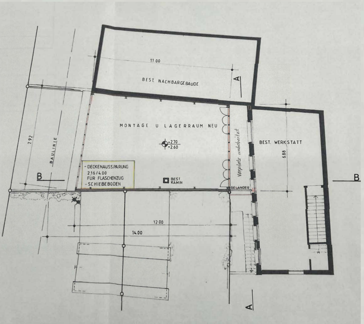
GRUNDRISS OBERGESCHOSS
