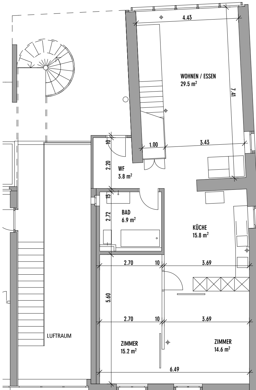
01 OBERGESCHOSS BURGGASSE 26, MUTTENZ
