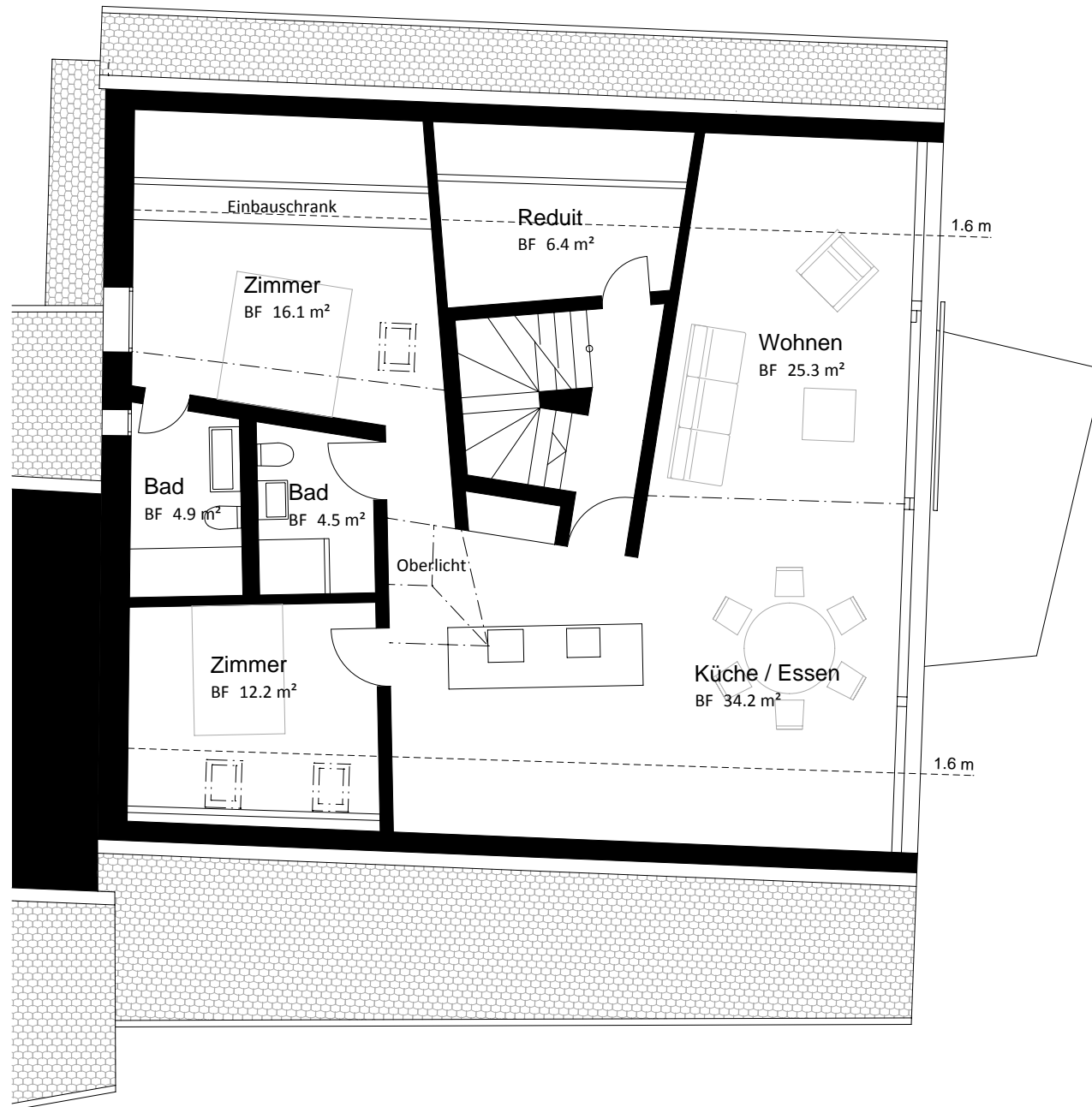
Dachgeschoss, M 1:100
