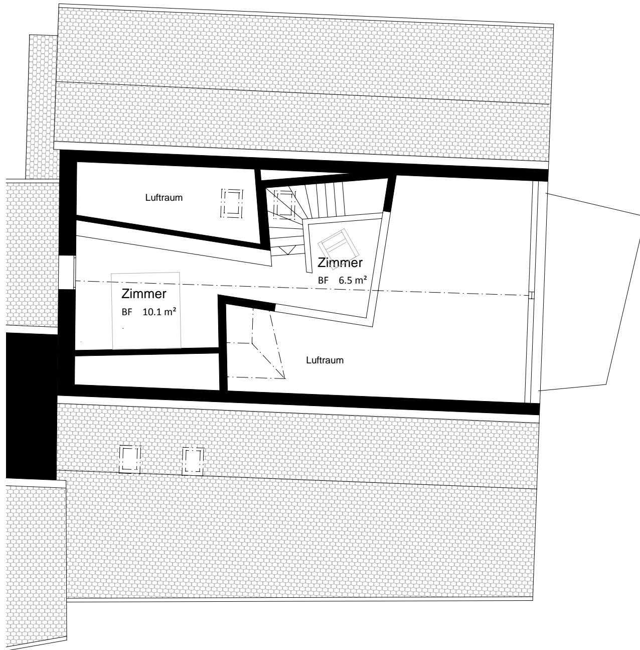
Galerie, M 1:100
