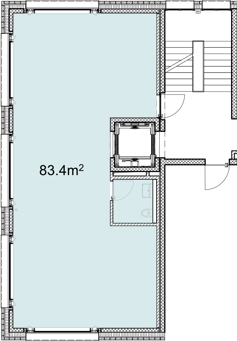
3.Obergeschoss
