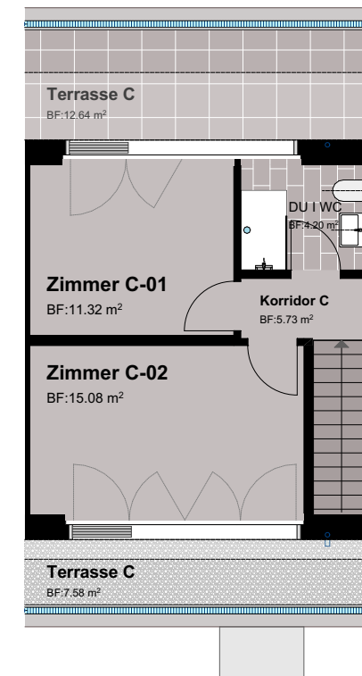
Obergeschoss
