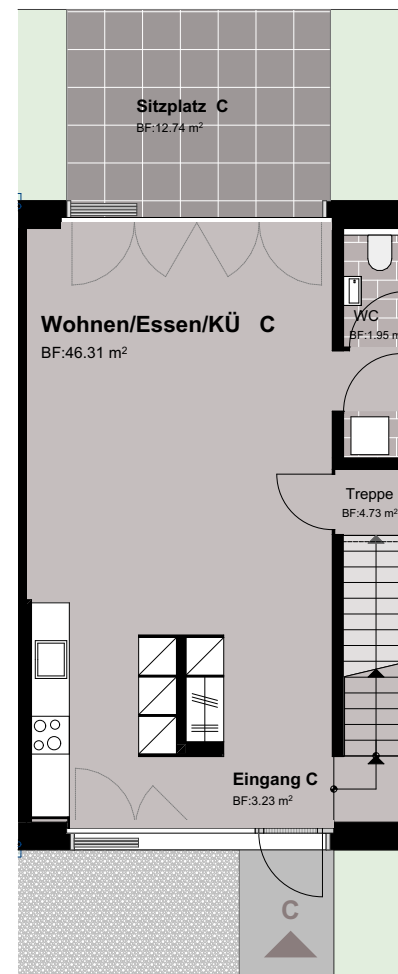
Erdgeschoss
