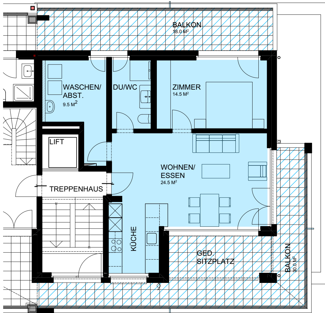
2 1 / 2 ZIMMER-WOHNUNG 2. OBERGESCHOSS WOHNFLÄCHE 63.0 M 2
