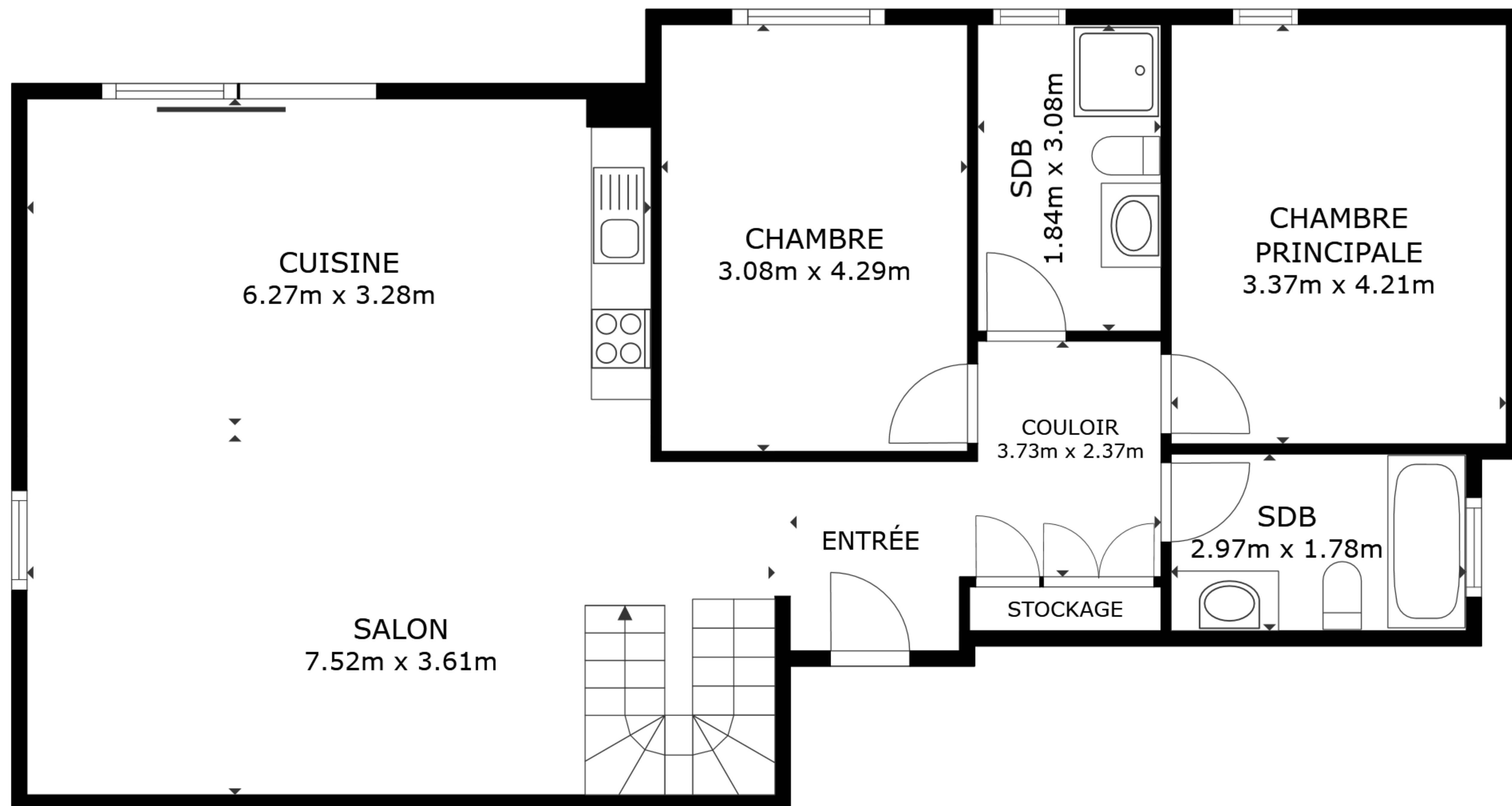
ÉTAGE 1
