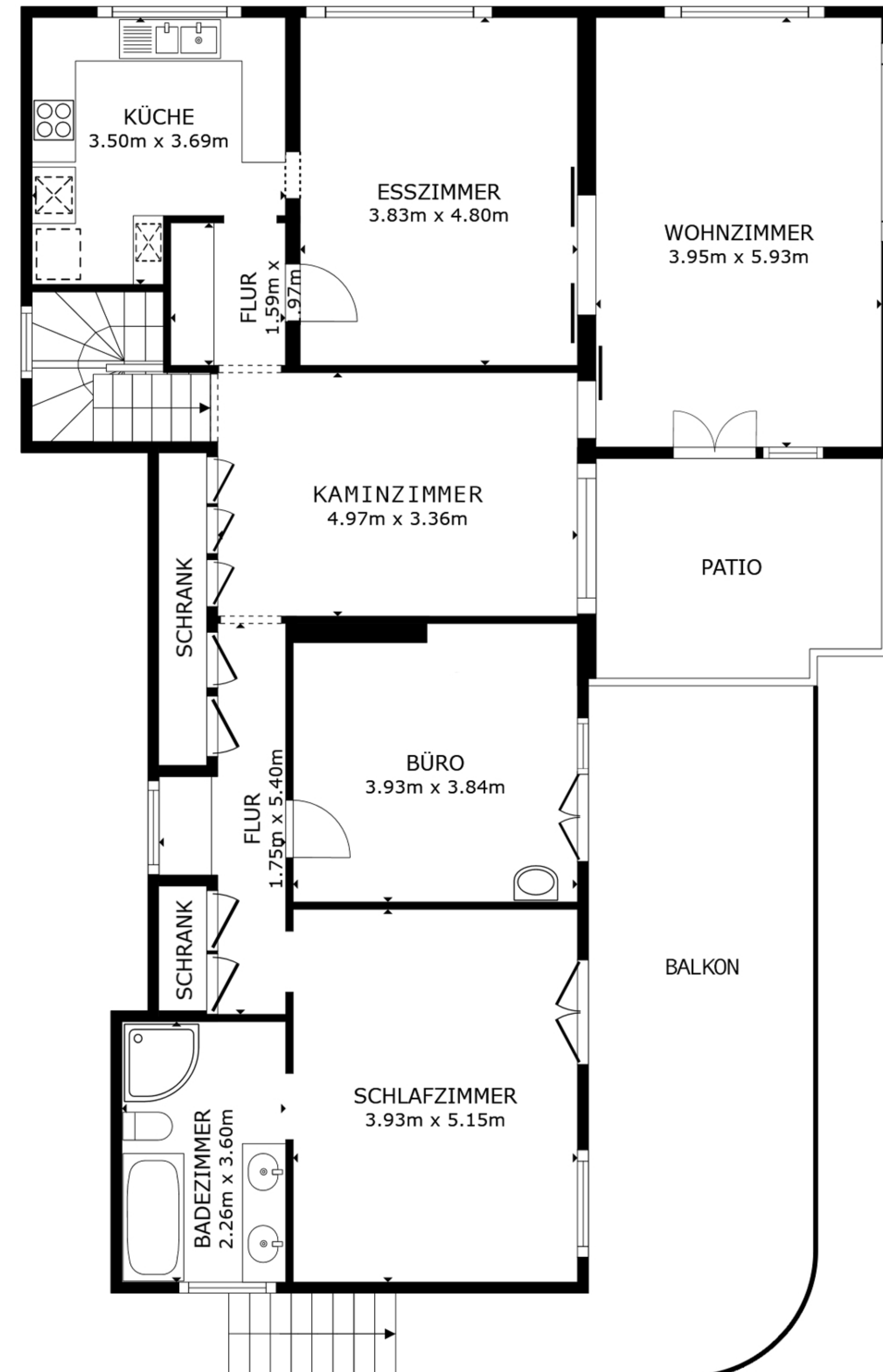
STOCKWERK 2
